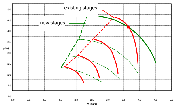
Figur 3: Einfluss der neuen Stufenauslegung auf das Betriebsverhalten eines mehrstufigen Verdichters. Unten: \pi -V-Kennfeld (Druckverhältnis-Volumenstrom); Oben: P-V-Kennfeld (Leistung-Volumenstrom).
