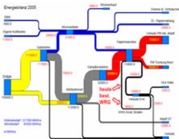
Figur 4: Energieflussdiagramm.
