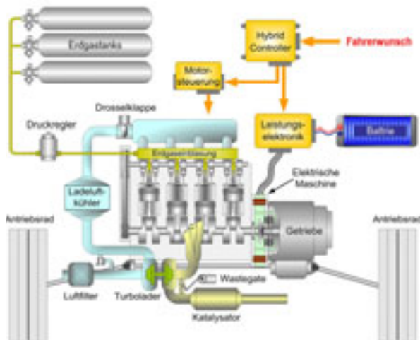
Figur 4: Geplanter Aufbau des Antriebsstrangs für das Projekt CLEVER.
