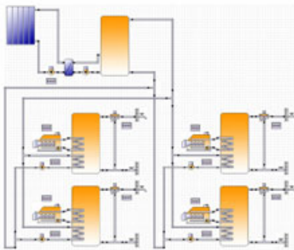
Figure 6 : un système solaire pour le collectif, typique de l'Espagne, avec préparation décentralisée d'eau chaude sanitaire, que la version Designer de Polysun 4.0 peut désormais définir et simuler (source : SPF).
