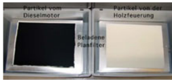
Figur 5: Partikel von Dieselmotor und Holzfeuerung auf beladene Planfilter.
