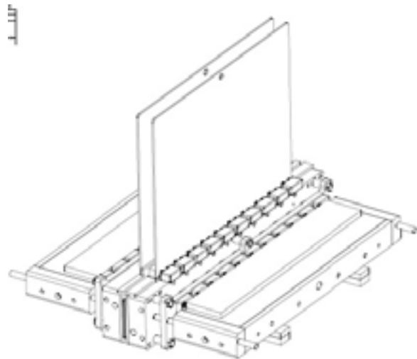
Figur 9: Modellbrennstoffzelle zur lokalen Gasanalyse [11].
