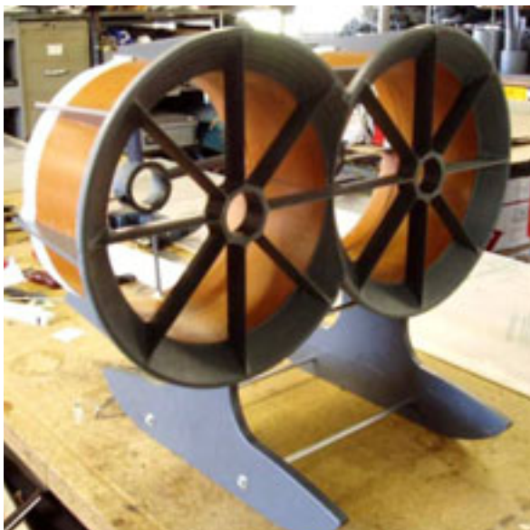
Figur 3: Modell des doppelten «Unterwasser-Drache» an der EPFL, hier noch ohne Laufrad. (Bild: Gresham SàRL / EPFL).
