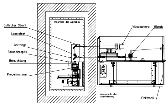
Figur 3b: Schematischer Aufbau der LA-ICP-MS.
