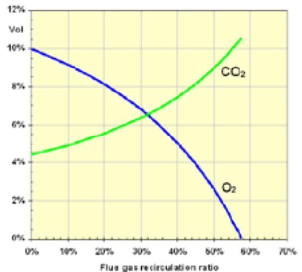
Figur 7: Einfluss der Abgasrezirkulation auf den Gehalt an \text{CO}_2 und \text{O}_2 im Abgas.
