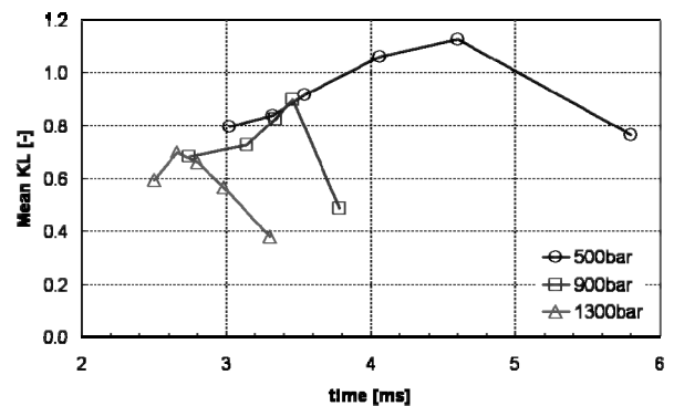
Figur 6: Gemittelte KL-Faktoren mit Diesel bei verschiedenem Einspritzdruck.
