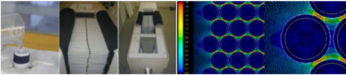
Figure 8 : un nouveau caisson expérimental avec 0.25 m 3 de stock a été élaboré et utilisé ici avec la variante de tubes à eau et modélisation CFD d'un coolshift stock diffusif en tubes (source : CUEPE, CMEFE).
