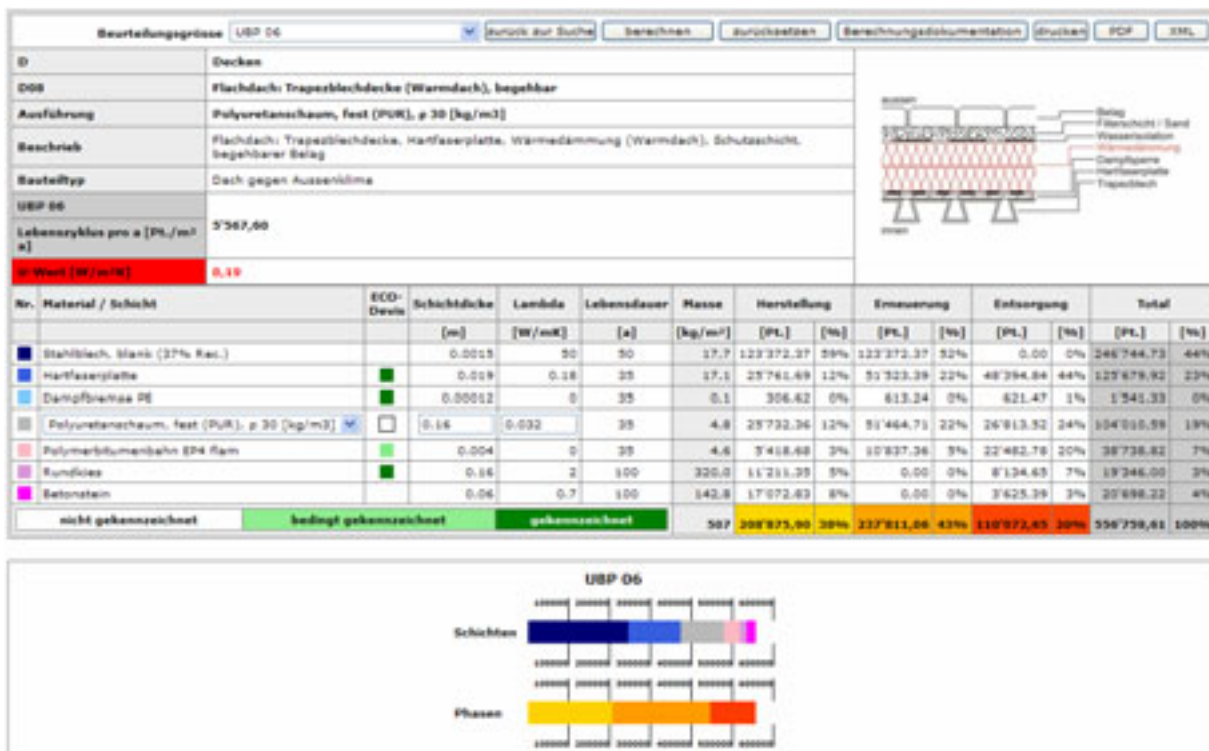
Figur 3: Das Beurteilungsschema enthält einerseits die entsprechenden Bauteilinformationen (Beschreibung, U-Wert etc.) sowie den Schichtaufbau (Materialisierung) des Bauteils.
