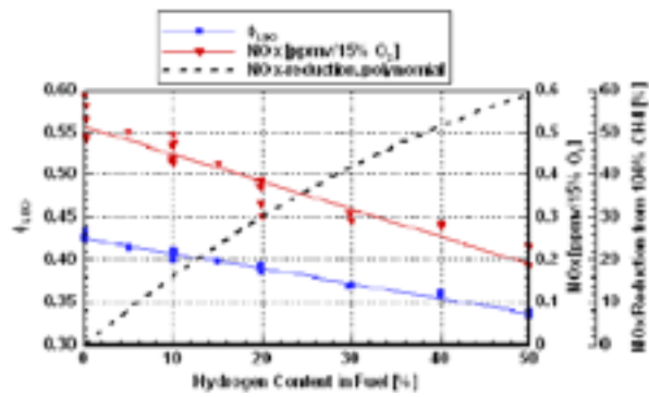
Figur 4: Löschgrenzen \Phi_{LBO} und minimale NO_x -Emissionen von Methan/Wasserstoff-Vormischflammen ( T_{Luft}=673\text{ K} , 5 bar, 40 m/s, Turbulenzgitter g365,xg10).
