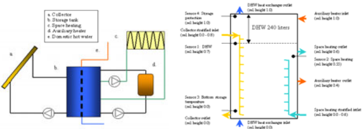
Figure 9 : simplification extrême d'un système solaire combiné, avec drain back et avec une cuve sans pression et avec un système d'injection directe dans le chauffage à débit variable ; le système est plus simple et plus performant ; il faut encore le tester en pratique (source : SPF) [24].
