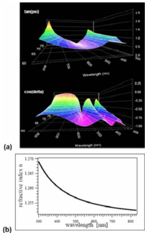
Figure 5 : détermination par ellipsométrie de l'indice de réfraction du film de nano-composite Mg-F-Si-O : (a) mesures ; (b) indices de réfraction prédits par la simulation (source : LESO PB).
