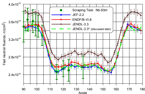
Figur 1: Schnelle Neutronenfluenz (> 1MeV) ermittelt mit Monte-Carlo unter Benutzung von 3 nuklearen Bibliotheken und Vergleich mit den Messdaten der Kratzproben.
