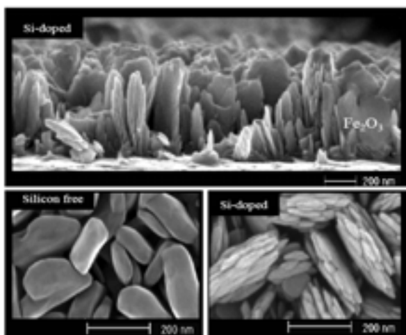
Figur 11: Morphologie von undotierten und durch Ultraschallspray Pyrolyse (USP) siliziumdotierten \text{Fe}_2\text{O}_3 -Photoanoden. Si-Dotierung und ein Depositionsverfahren welches eine möglichst grosse Gesamtoberfläche erzeugt sind massgebend für eine signifikante Effizienzsteigerung [13].
