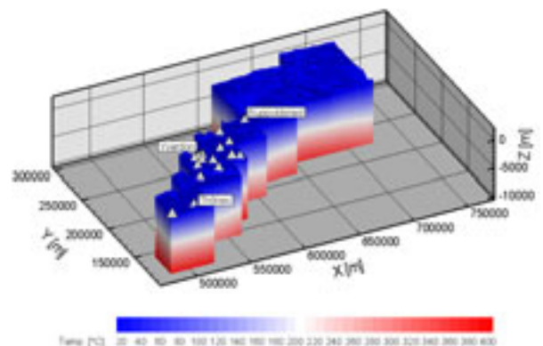
Figure 3: Résultats du calcul de la température en 3D des modèles diffusifs de Genève, WS1 à WS4, Soleure, Bâle, NOS I à NOS III, et AG_ZH.
