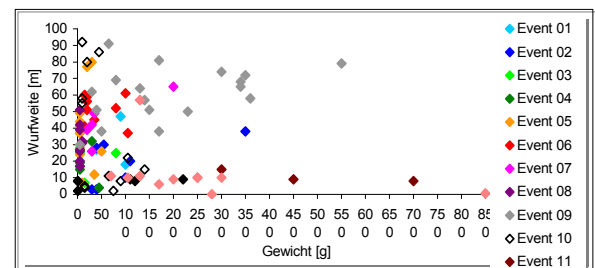
Figur 6: Darstellung der gefundenen Eisstücke am Standort Gütsch, Wurfweite nach Gewicht.
