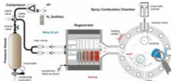
Figur 3: Schema der gesamten Versuchseinrichtung mit Darstellung der Aufheizphase.
