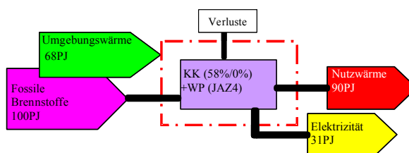
Figur 1: Energiefluss der Kombination von Kombi-Kraftwerken (KK) und Wärmepumpen (WP). Aus 100% fossiler Energieträger können Nutzwärme mit einem Effizienzgrad von 90%, und gleichzeitig elektrische Energie mit einem Effizienzgrad von 31%, bereitgestellt werden. Das Kombikraftwerk hat einen elektrischen Wirkungsgrad von 58% mit 0 % Abwärmenutzung und die Jahresarbeitszahl der Wärmepumpe beträgt 4.0.
