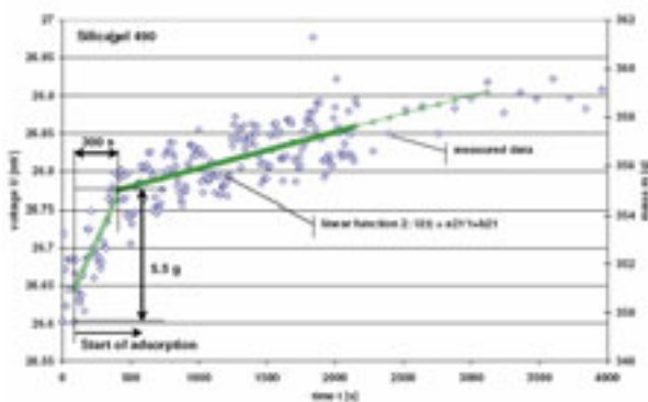
Figure 10 : adsorption d'eau dans un lit de «silicagel 490» ; on observe dès apparition de la saturation une nette diminution de gain ; la saturation a lieu après 300 s contre 400 s pour la «zéolithe 13X» (source : SPF).
