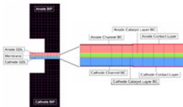
Figur 6: Simulationsgebiet: Kleinste repetitive Einheit der Testzelle (links) und vergrößerter Ausschnitt der MEA (rechts) mit Randbedingungen [6].
