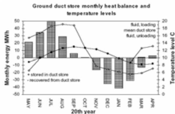
Figure 7 : exemple de sortie du logiciel Bridgesim pour la simulation d'un pont dégivré par un stock saisonnier diffusif. Le bilan et les températures de la 20 e année de fonctionnement (source : LEEE).
