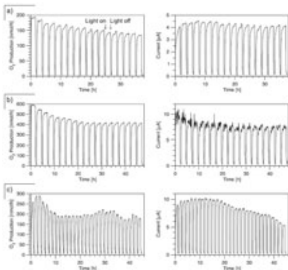
Figur 14: O_2 -Produktion und Photostrom versus Zeit für drei verschiedene Photoanoden. a) AgCl-Elektrode, b) Zeolith-A-Monoschicht modifiziert mit AgCl, c) Zeolith-L-Monoschicht modifiziert mit AgCl [16].
