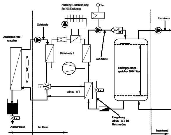
Figur 2: Schema der untersuchten Wärmepumpen-Anlage mit dem witterungsgeführten Ladewasserstrom. Die Regulierung geschieht durch die Elemente in der Mitte oben, wo die Umgebungstemperatur T_u auf den Regler der Umwälzpumpe im Ladekreis einwirkt.
