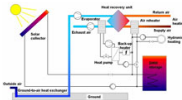
Figur 3: Untersuchtes Kompaktgerät mit den Funktionen Heizen, Wärmerückgewinnung, und Brauchwasserbereitung.
