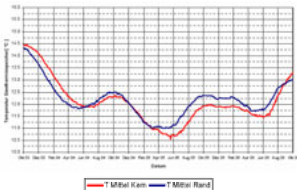
Figure 13 : évolution de la température du stock du bâtiment de la SUVA entre octobre 2003 et octobre 2005 (source : PB).
