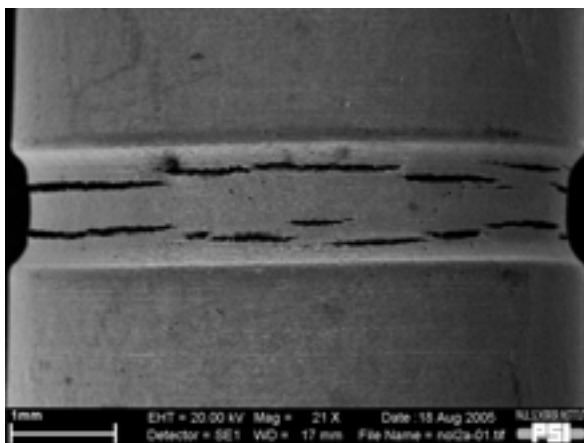
Figur 1: Spannungsrissskorrosions-Risse in gekerbter Rundzugprobe aus rostfreiem Stahl (Quelle: PSI).
