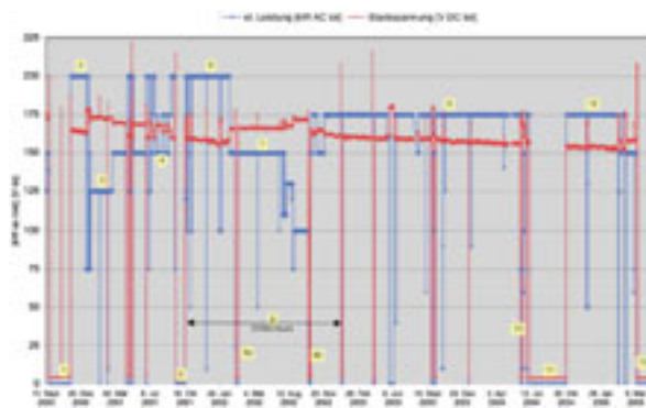
Figur 18: Leistungs- (Stufen) und Spannungsverlauf (variable Kurve) der ONSI-Zelle über die ganze Betriebszeit von 36'000 h [28].
