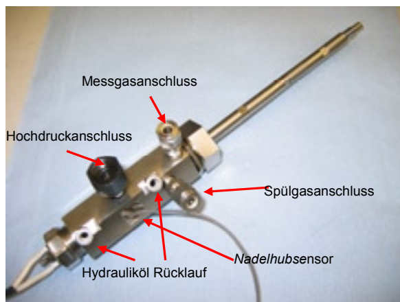
Figur 8: Zusammengebaute Entnahmesonde mit Bezeichnung der erkennbaren Anschlüsse.
