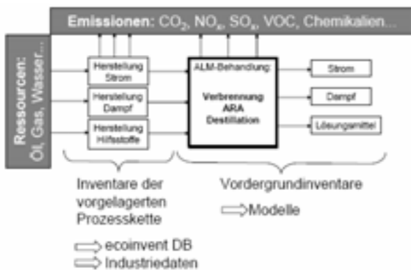
Figur 9: Bilanzierungsgrenze - Sachbilanz.
