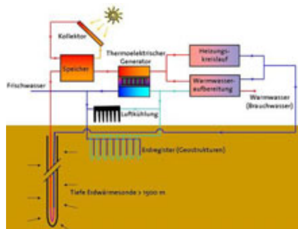
Figur 2: Schema einer thermoelektrischen Energiekonversion im Gebäude (ETH Zürich).
