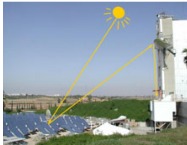
Figur 3: Experimenteller Aufbau des 300 kW Pilotreaktors (oben) in der «Beam-Down»-Solaranlage am Weizmann Institute of Science, Rehovot, Israel (unten).
