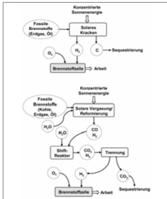
Figur 4: Schema von zwei solaren Hybridprozessen für die Dekarbonisierung von fossilen Brennstoffen zur Herstellung von Wasserstoff und Strom. Fossile Brennstoffe dienen als Rohmaterial und die konzentrierte Sonnenenergie als Quelle für die Hochtemperatur-Prozesswärme. Die Vorteile dieser Prozessführung sind dreifach: 1) CO 2 -Emissionen werden vermieden; 2) die gasförmigen Produkte werden nicht durch Verbrennungsnebenprodukte kontaminiert; 3) der Heizwert des fossilen Brennstoffs wird erhöht [11].
