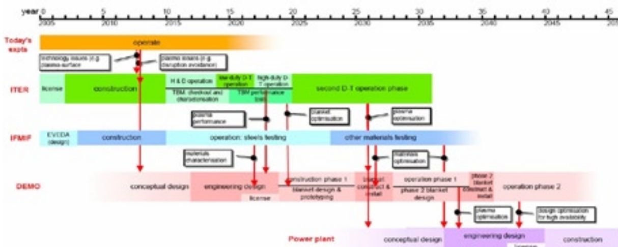
Figure 2 : la planification du projet ITER prévoit une durée de construction d'environ 10 ans, qui a maintenant débuté, suivie d'une durée d'utilisation d'environ 20 années répartie sur deux phases. Ces durées s'inscrivent dans une planification à long terme, passant par DEMO, jusqu'au démarrage des premiers réacteurs à fusion.
