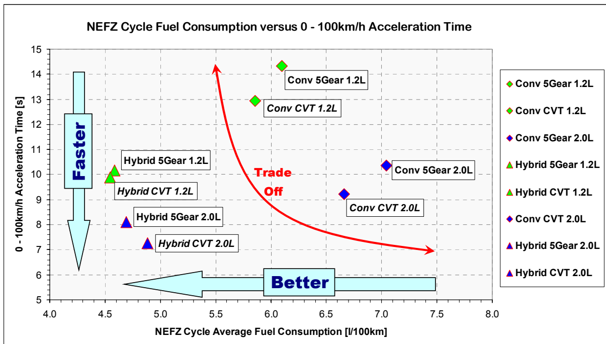
Figur 9: Trade-off zwischen Treibstoffverbrauch und Beschleunigungszeit von Null auf 100 km/h.
