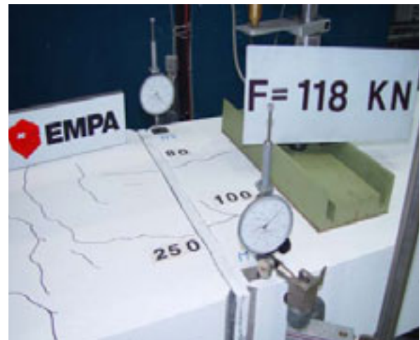
Figur 11: Beim Prüfkörper TTE «Q» D18 MM wurde eine maximale Querkraft von Q = 124.2 \text{ KN} erreicht. Das maximale Moment betrug M = 36.63 \text{ KNM} .
