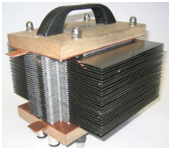
Figur 22: Der in Zusammenarbeit FH Biel und CeKa AG im KTI Projekt IPHoS entwickelt, luftgekühlte PEFC-Stapel [22].
