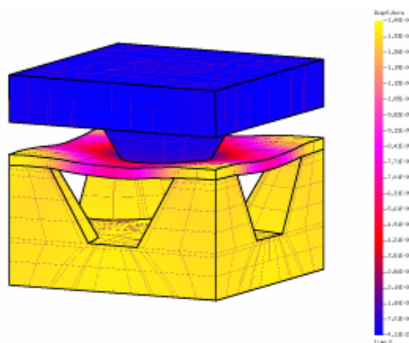
Figur 5: Repetitives Element eines Hexis SOFC Stacks geprüft unter externer Last. Das 3D Seses FE-Model wird verwendet um die räumlich gemittelten, mechanischen Eigenschaften zu berechnen [5].
