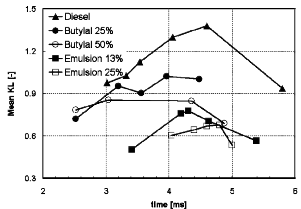
Figur 7: Gemittelte KL-Faktoren bei verschiedenen Treibstoffen.
