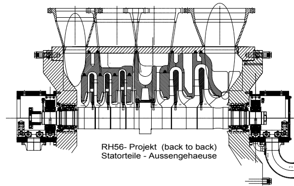
Figur 2: Repräsentativer Verdichterschnitt.
