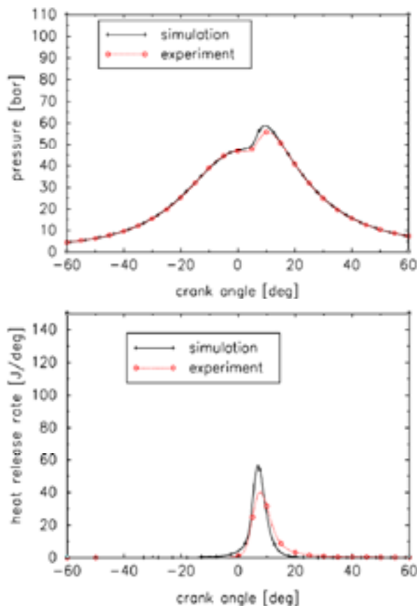
Figur 4: Vergleich des berechneten Druckverlaufs (links) bzw. der Wärmefreisetzung (rechts) mit den Messungen für Betriebspunkt 1 ( n = 1200 U/min, 20 Temperaturzonen, 10 Lambdazonen, \lambda = 3.8 , \sigma_T = 2.5 K, \sigma_\lambda = 0.05 , n-Butan, reduzierter Mechanismus, \alpha_{\text{scaling}} = 0.5 ).
