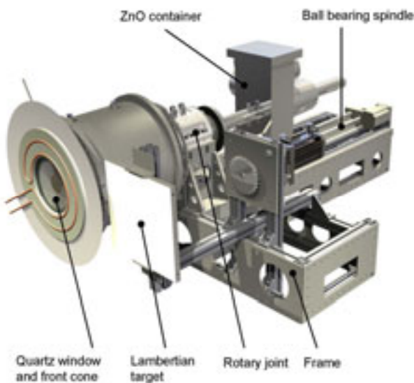
Figur 2: Experimenteller Aufbau des 10 kW Prototypreaktors im Hochfluss-Solarsimulator am PSI [10].
