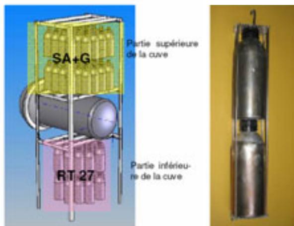
Figure 11 : 2 types de PCM introduits dans une cuve de système solaire combiné (SA+G = acétate de sodium avec poudre de graphite, RT27 = paraffine) et récipients utilisés (source : LESBAT).
