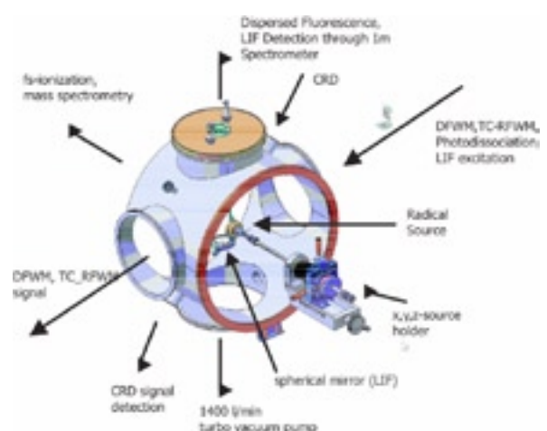
Figur 2: Versuchapparat für nichtlineare spektroskopische Messungen in einem Molekularstrahl.
