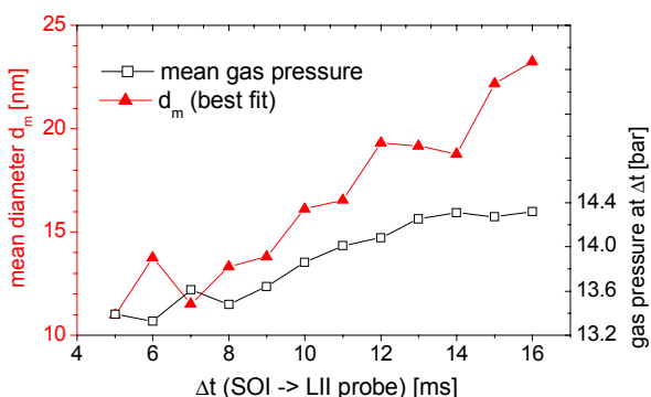
Figur 5: Zunahme der mittleren Partikeldurchmesser der Russteilchen (Dreiecke) und mittlerer Gasdruck (Quadrate) als Funktion der Zeit zwischen Einspritzbeginn und LII-Laserpuls.
