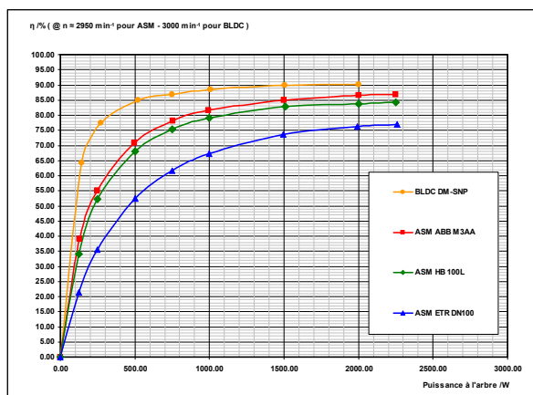
Figur 4: Wirkungsgrad-Verlauf eines Permanentmagnet-Motors (Typ: BLDC-DM-SNP) im Vergleich zu drei Asynchronmotoren unterschiedlicher Effizienzklassen (Circle Motor AG).
