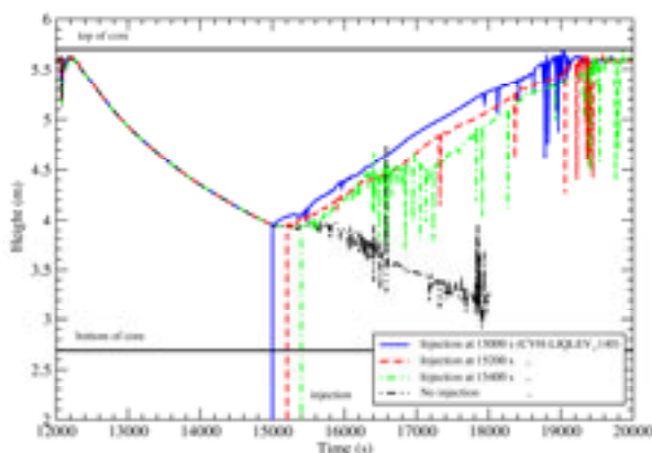
Figur 5: Zeitlicher Verlauf des Wasserpegels im Bereich des Reaktorkerns für drei verschiedene Startzeiten der Auffüllpumpe und für den Fall ohne Einspeisung
