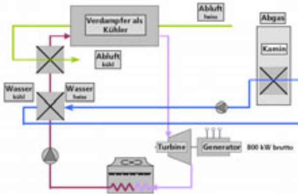
Figur 5: Schema des geplanten Prozesses zur Abwärmenutzung.
