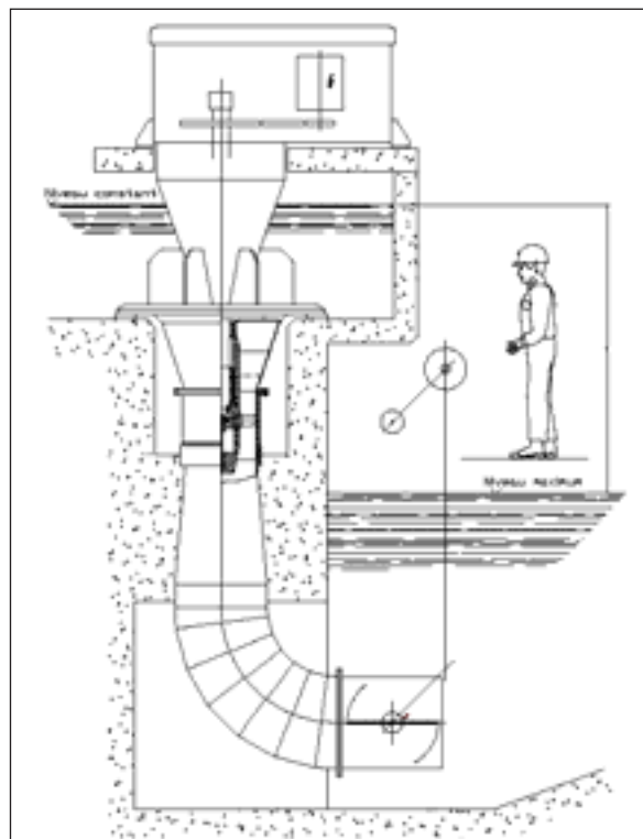
Figur 2: Niederdruckturbine aus dem Hause MHyLab; auf dieser Technologie aufbauend werden gegenwärtig die neuen Diagonalturbinen entwickelt. (Bild: MHyLab).
