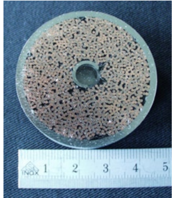
Figure 4 : section d'un câble supraconducteur (PSI).
