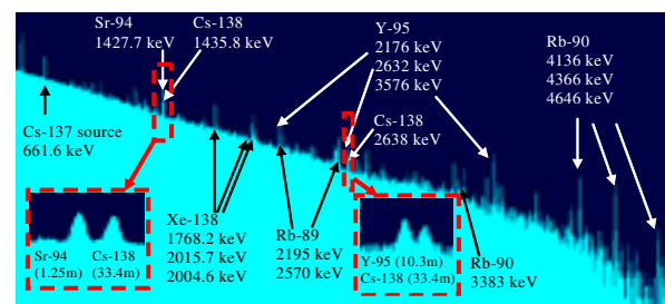
Figur 2: Typisches Gammaspektrum von 4% angereichertem UO_2 mit kurzlebigen Spaltprodukten, wie es im BR1-Reaktor in Mol gemessen wurde (Bestrahlungszeit 15 Min., Messzeit 10 Min., Bleifilter 4 cm).
