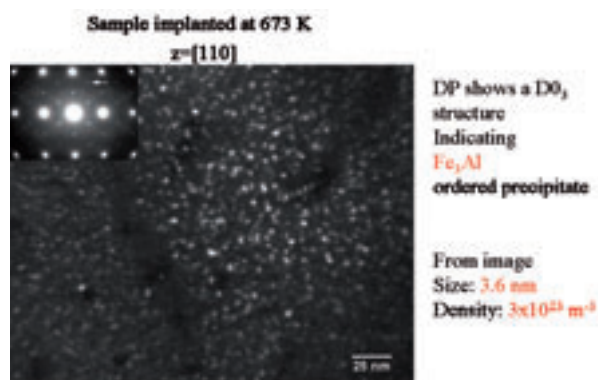
Figur 7: TEM Abbildung einer strahlungsinduzierten intermetallischen Fe 3 Al Ausscheidung in der ferritischen ODS-Legierung PM2000. Bestrahlungstemperatur 400°C. TEM Dunkelfeldabbildung mit Überstruktureflex (DP = Beugungsbild, D0 3 = zugeordnete Kristallstruktur).
