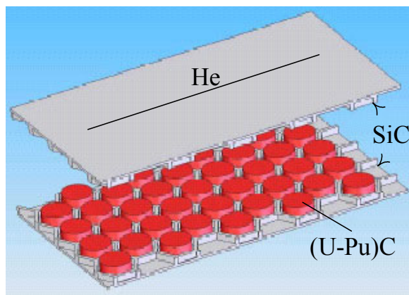
Figure 9a: GFR Brennelement (Platte).
