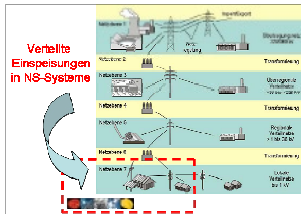
Figur 2: Überblick über den Einsatz von verteilten Einspeisungen in 400 V Niederspannungsnetzen (Quellen: VSE, Projekt VEiN).
