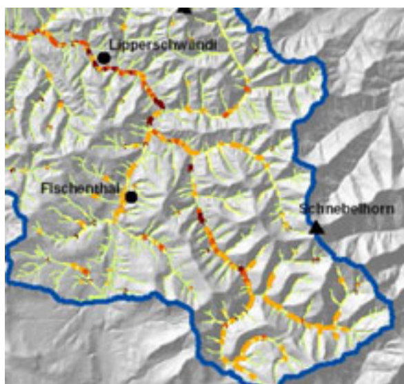
Figur 5: Digitales Geländemodell (oben) und, als Ergebnis der numerischen Potenzialberechnung, die Energiedichte der einzelnen Gewässerabschnitte im oberen Einzugsgebiet der Töss – je dunkler, desto höher das Potenzial. (Bilder: Uni Bern).
