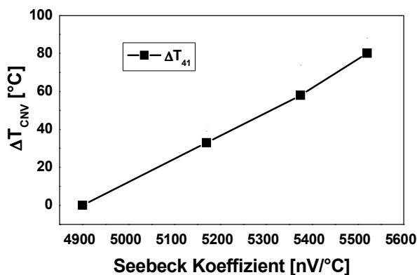
Figur 4: Verschiebung der Duktile-Sprödbbruch-Übergangstemperatur \Delta T_{CNV} als Funktion des Seebeck-Koeffizienten, gemessen an Charpy Kerbschlagproben aus dem Reaktordruckbehälterstahl JRQ.
