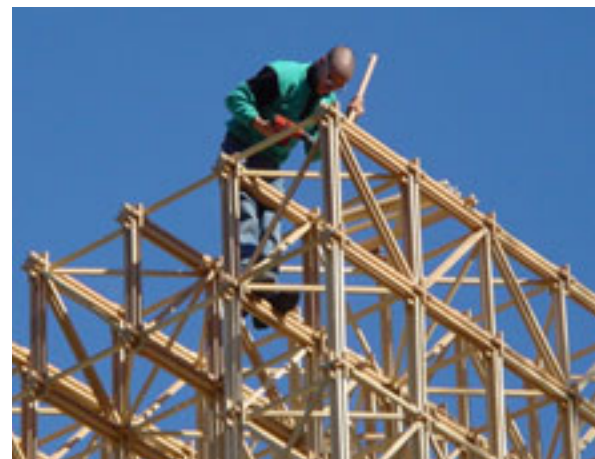
Figur 6: Das dreidimensionale Fachwerk aus Holzstäben und Holzknotten wird mit Zelluloseflocken ausgeblasen und bildet eine rundum wärmebrückenfreie Gebäudehülle für Wände, Boden und Dach (Bild: David Muspach).
