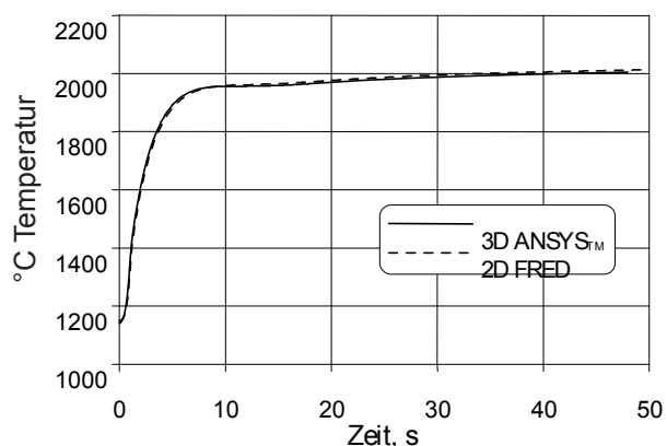
Figure 9b: Spitzen-Brennstofftemperaturen während eines UTOP-Unfalls berechnet mit den Modellen FRED (2D) und ANSYS TM (3D).
