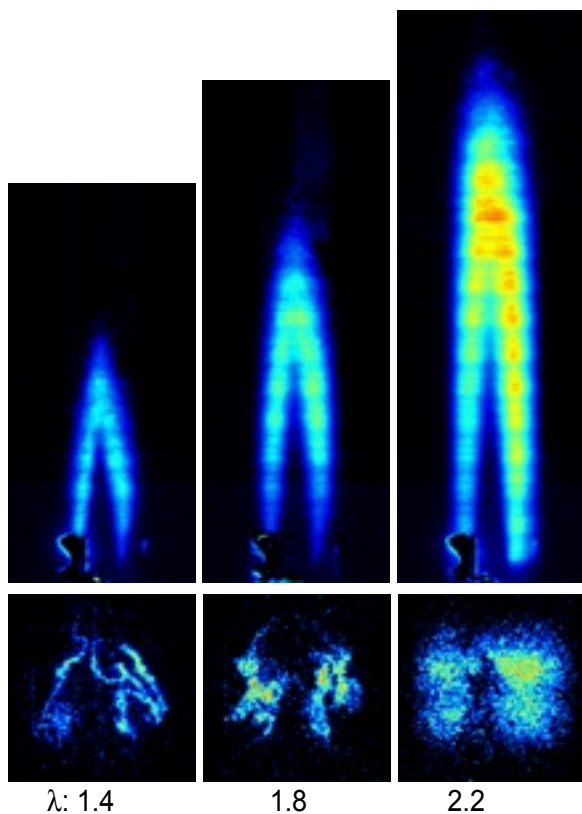
Figur 8: Gemittelte (oben) und Einzelpuls (unten) \text{CH}_2\text{O} «laser induzierte Fluoreszenz»-Bilder einer turbulenten mageren Vormischflamme ( T_{\text{Luft}}: 773 \text{ K} ) für verschiedene Luftzahlen \lambda .
