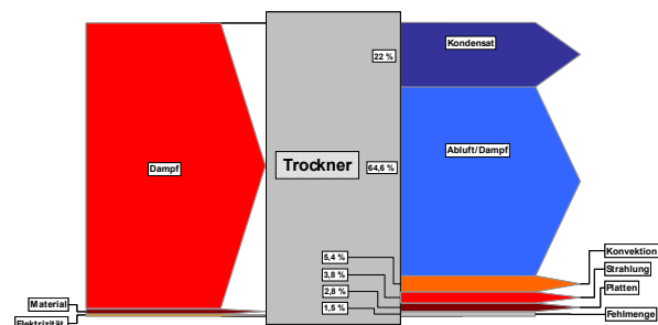
Figur 8: Energieflüsse im Trockner.
