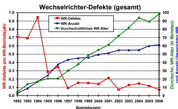
Figur 4: Wechselrichter-Defekte pro Wechselrichter-Betriebsjahr (Bildquelle: FH Burgdorf).
