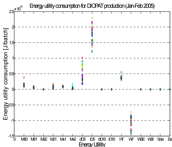
Figur 1: Variabler Energieverbrauch verschiedener Batches.
