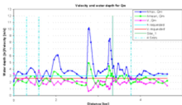
Figur 4: Für den Einsatz von UEK-Turbinen müssen die Wassertiefe (oberste Kurve) und die Strömungsgeschwindigkeit (unterste Kurve) genügend hoch sein. (Bild: Gresham SàRL / EPFL).
