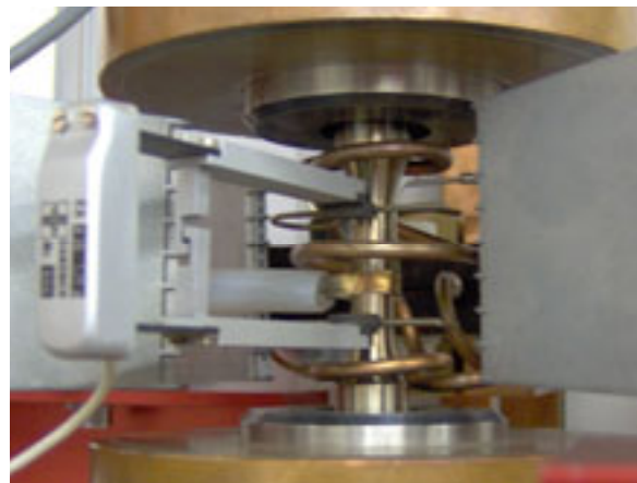
Figur 2: Versuchseinrichtung für thermomechanische Ermüdung (Quelle: PSI).
