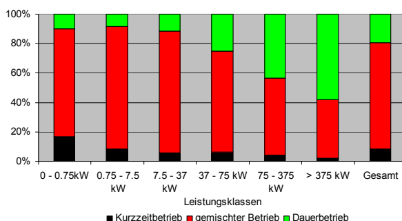
Figur 8: Verteilung der Betriebszustände in Abhängigkeit von der Leistungsklasse. Die Anteile beziehen sich gesamthaft auf rund 16'000 Motoren, für die entsprechende Informationen aus der Industriebefragung zur Verfügung stehen (basic).
