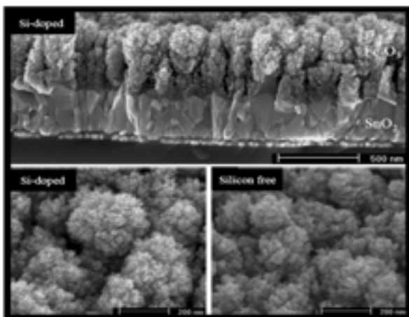
Figur 12: Morphologie von durch atmosphärische chemische Dampfdeposition (APCVD) siliziumdotierten und undotierten \text{Fe}_2\text{O}_3 -Photoanoden. Das angewendete Verfahren führt zu einer stark vergrösserten aktiven Oberfläche damit zu einer deutlichen Effizienzsteigerung [13].
