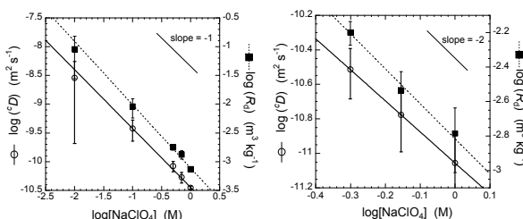
Figur 6: Logarithmische Darstellung der Abhängigkeit von ^{\circ}D und R_d für ^{22}\text{Na} (links) und ^{85}\text{Sr} (rechts) in kompaktiertem Montmorillonit von der Salzkonzentration in der externen Flüssigkeit, welche sich im Kontakt mit der Tonprobe befindet.
