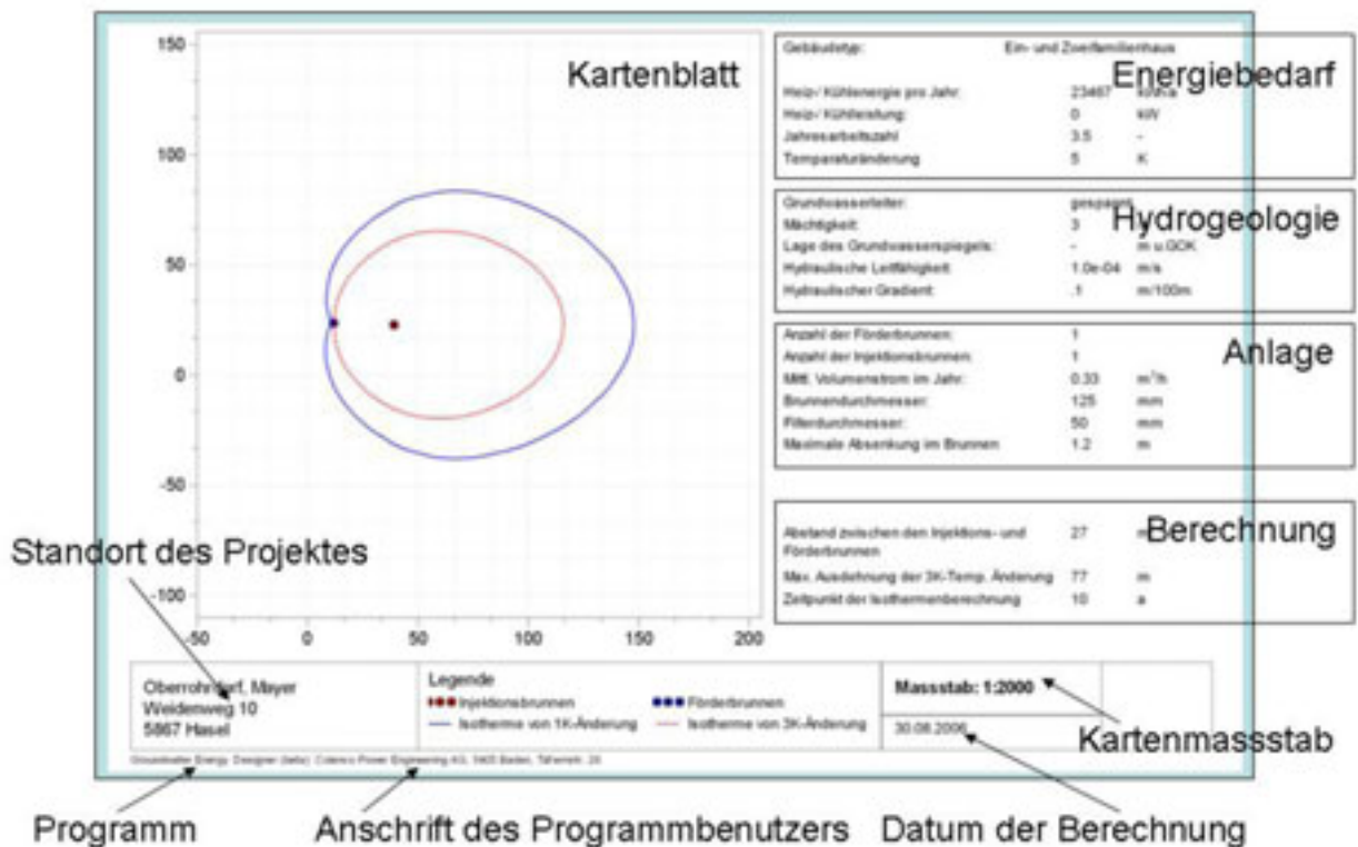
Figur 1: Groundwater Energy Designer: grafische Präsentation der Ergebnisse.
