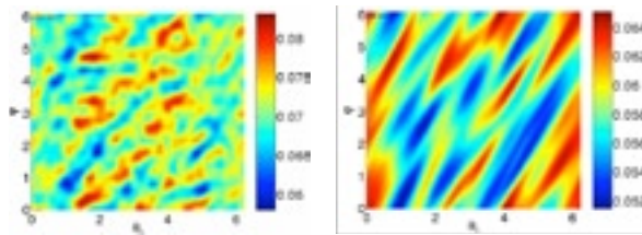
Figure 3 : détails de la turbulence simulée sur une surface magnétique. À gauche, les perturbations se noient dans le « bruit numérique ». À droite, une méthode de filtrage des perturbations dans la direction des lignes de champ magnétique a permis d'éliminer ce comportement non physique (in : CRPP Annual Report 2005, p. 31).
