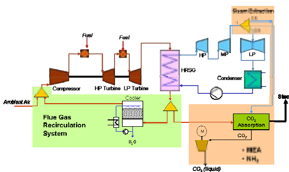
Figur 6: Schema eines Gas- u. Dampfturbinen-Prozesses mit Abgasrezirkulation und \text{CO}_2 -Abscheidung.
