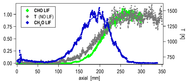
Figur 9: Normierte Profile von \text{CHO} , \text{CH}_2\text{O} LIF Signalen und der Temperatur in der Flammenfront einer mageren turbulenten Vormischflamme ( \lambda = 2.0 ).
