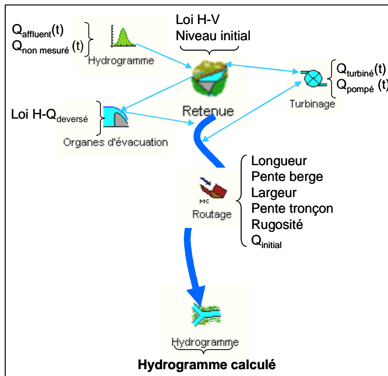
Figure 3 : Schématisation des données nécessaires pour la modélisation dans Routing System
