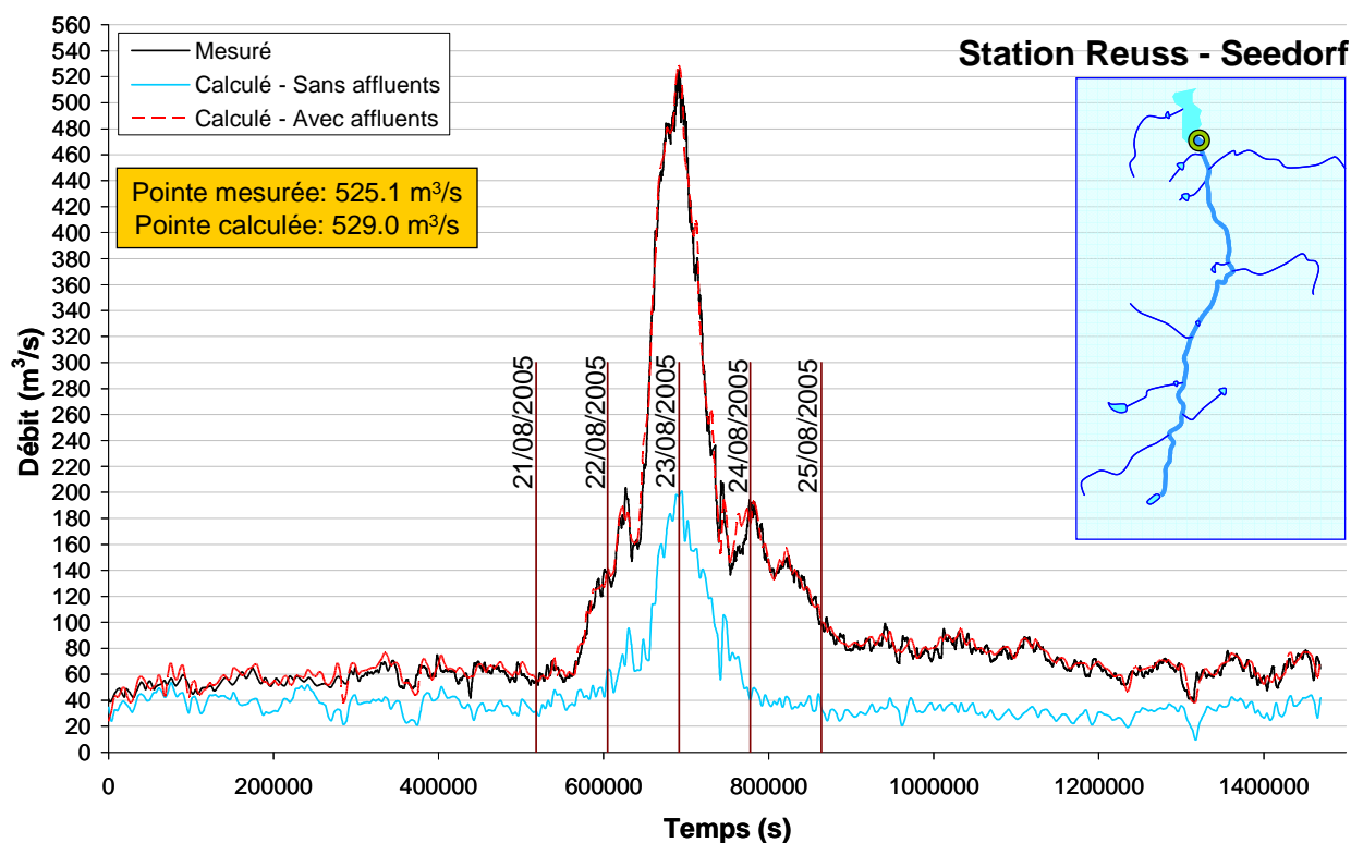
Figure 23 : Hydrogramme mesuré (en noir) et calculé (en rouge) à la station de Seedorf, sur la Reuss
