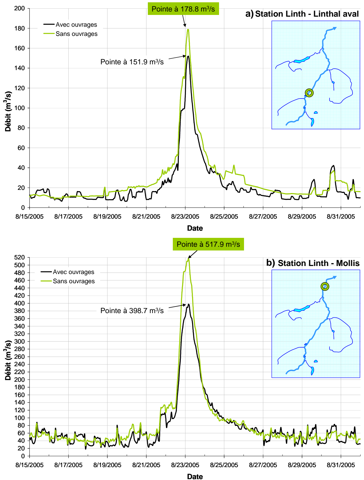
Figure 37 : Hydrogramme actuel avec ouvrages (en noir) et naturel sans ouvrages (en vert) au Linthal, en aval du baddin du Linthal (a) et à la station de Mollis (b) sur la Linth
