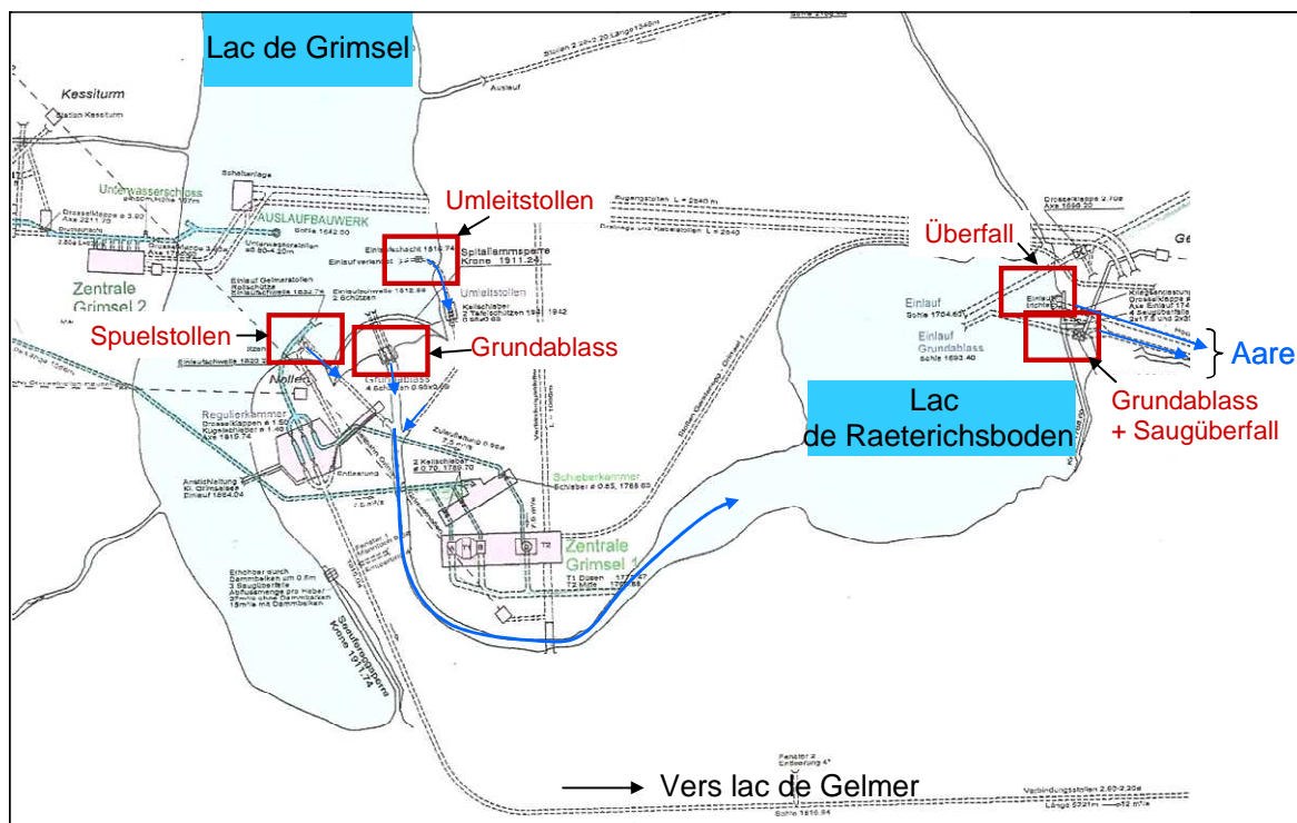
Figure 16 : Localisation des organes d'évacuation simulés dans le modèle numérique de l'Aare avec ouvrages
