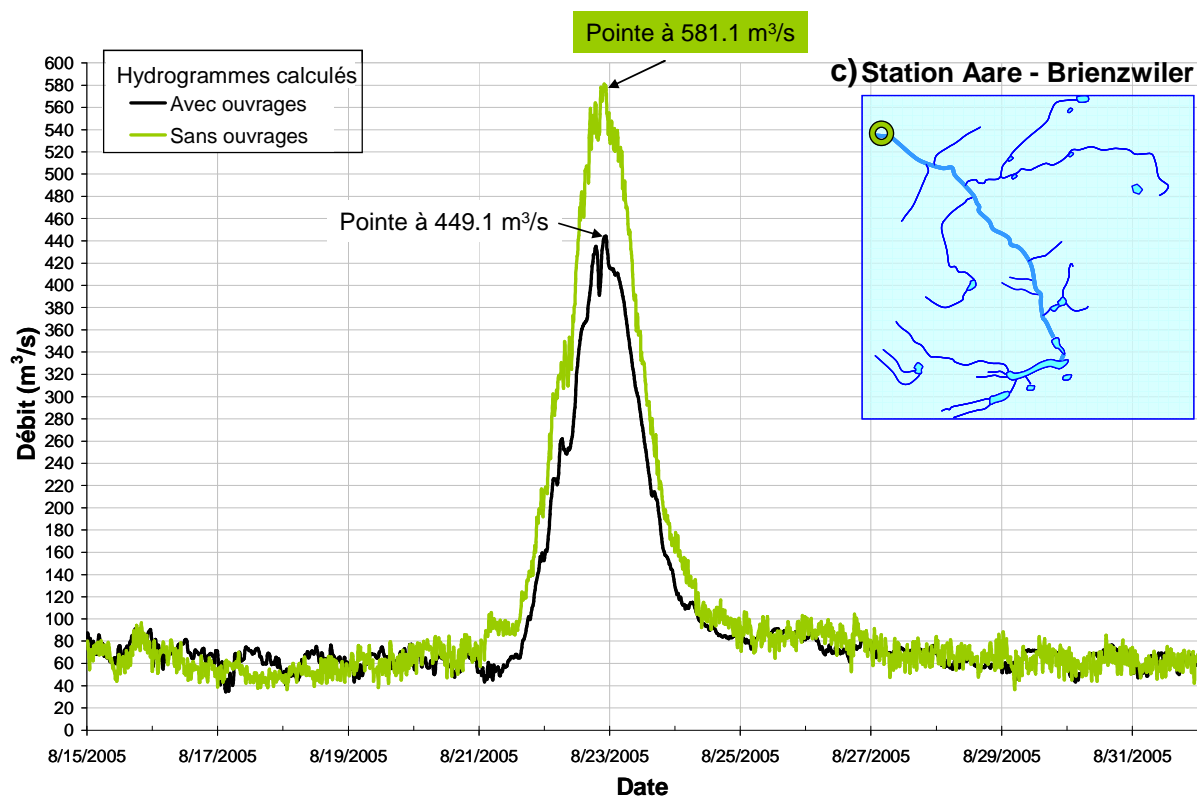
Figure 34 : Hydrogramme actuel avec ouvrages (en noir) et naturel sans ouvrages (en vert) de l'Aare à Guttanen (a), à la jonction avec l'Urbachwasser (b) et à Brienzwiler (c)
