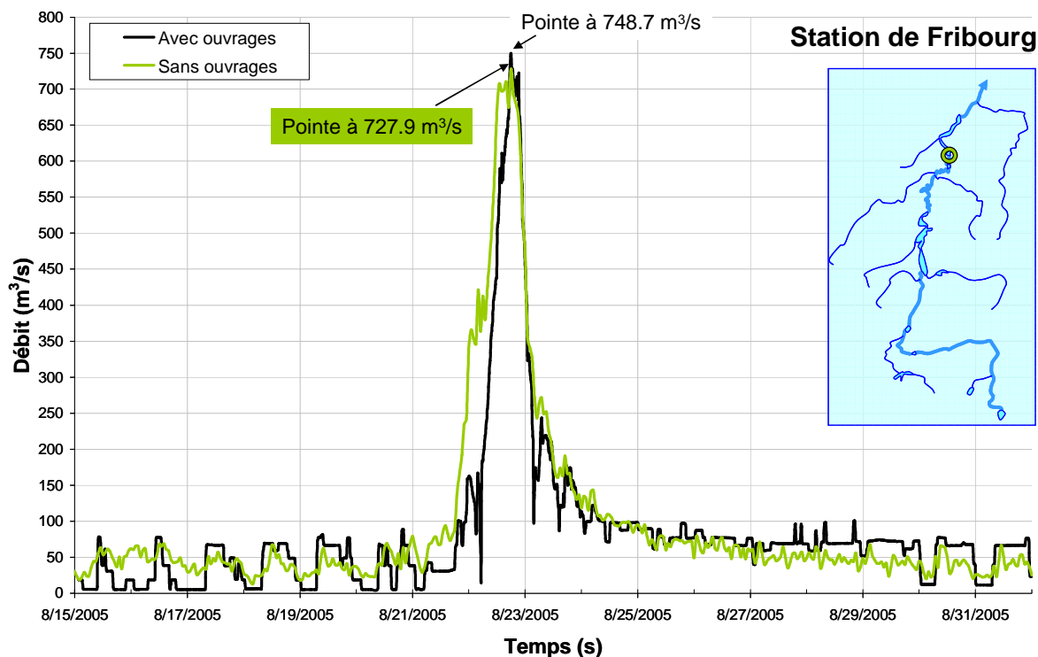
Figure 32 : Hydrogramme actuel avec ouvrages (en noir) et naturel sans ouvrages (en vert) à la station de Fribourg sur la Sarine
