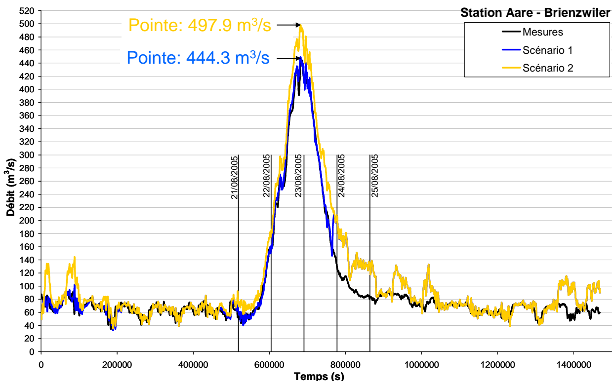
Figure 19 : Hydrogramme de la crue d'août 2005 mesuré (en noir), calculé-scénario 1 (en bleu) et calculé-scénario 2 (en orange) à la station de l'Aare-Brienzwiler – Avec ouvrages d'accumulation
