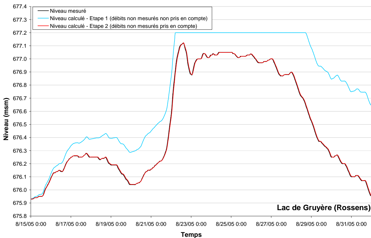
Figure 9 : Calage du niveau de la retenue de Rossens (lac de Gruyère) – Débit de vidange de fond non pris en compte (courbe bleu)
