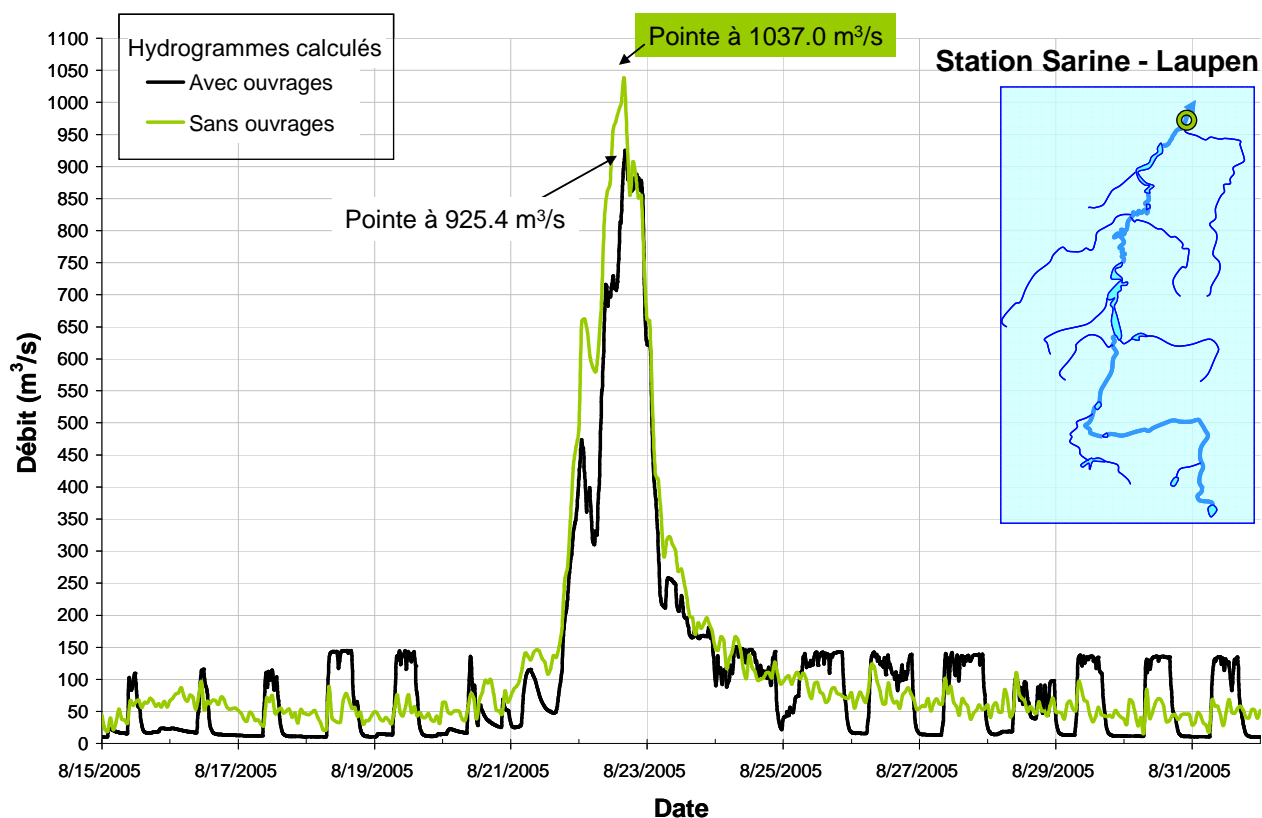
Figure 31 : Hydrogramme actuel avec ouvrages (en noir) et naturel sans ouvrages (en vert) à la station de Laupen sur la Sarine
