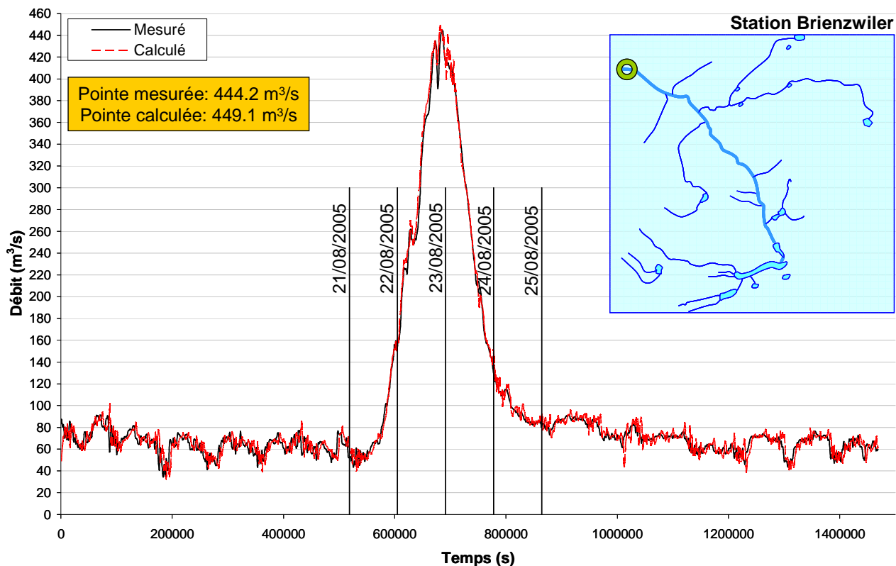
Figure 15 : Hydrogramme mesuré (en noir) et calculé (en rouge) à la station de Brienzwiler, sur l'Aare
