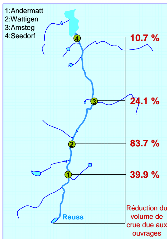
Figure 40 : Réduction locale du volume de la crue grâce aux ouvrages d'accumulation le long de la Reuss jusqu'à Seedorf du 21 août 2005 (0 h) au 24 août 2005 (24 h)
