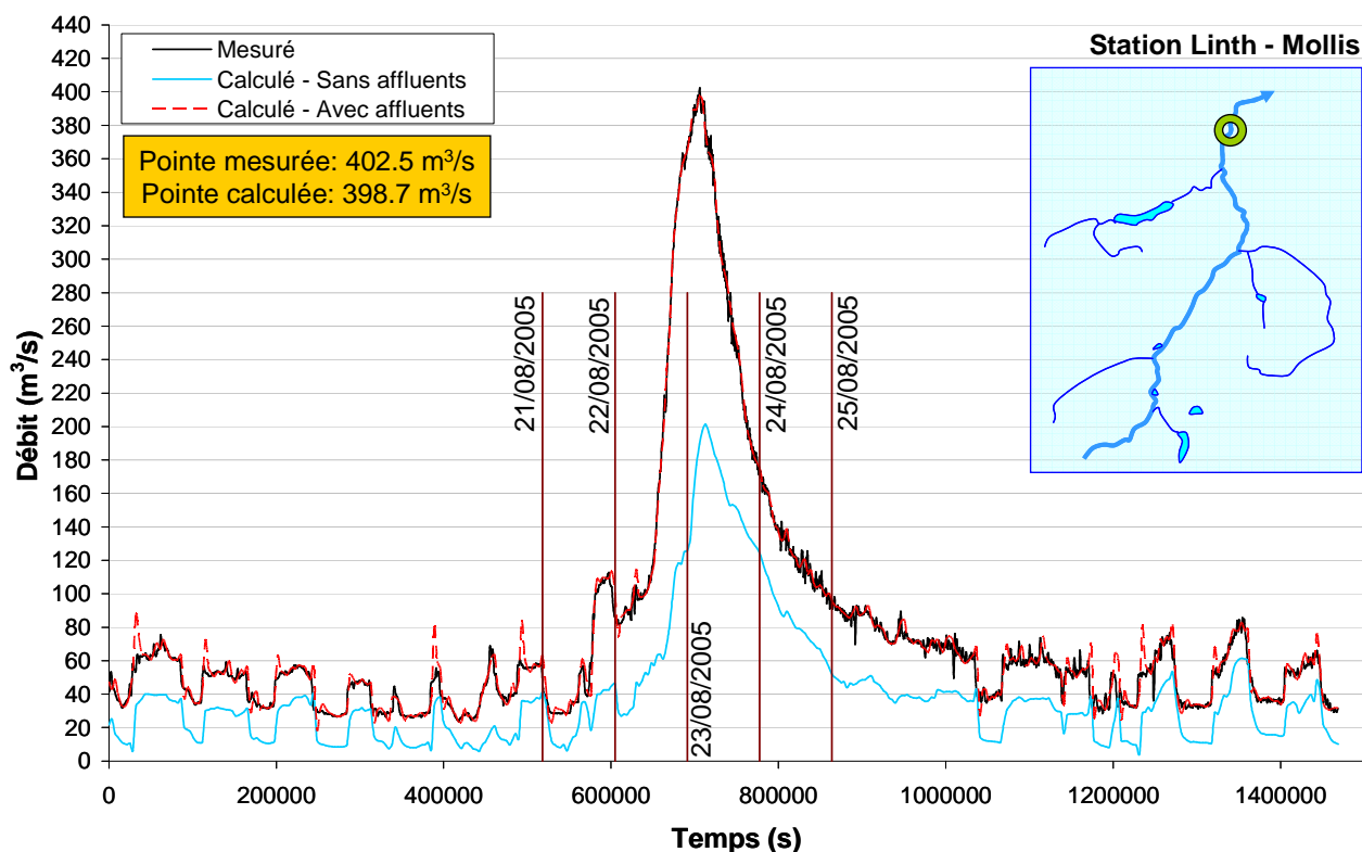
Figure 26 : Hydrogramme mesuré (en noir) et calculé (en rouge) à la station de Mollis, sur la Linth
