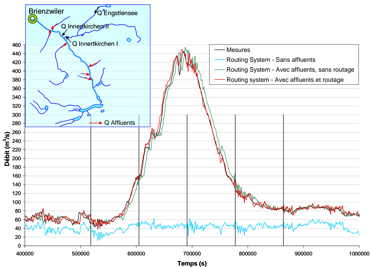
Figure 7 : Hydrogramme calculé avec Routing System à Brienzwiler (Aare)
