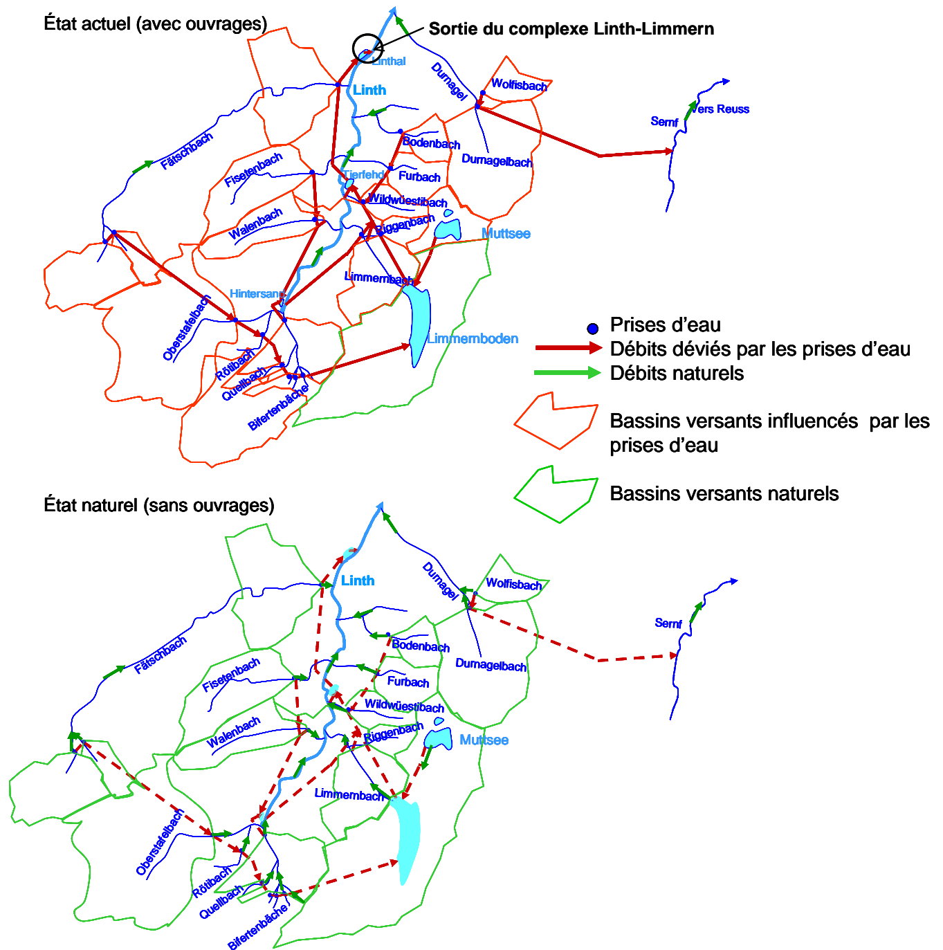
Figure 30: Définition des sous-bassins versants artificiels (en rouge) avec ouvrages et naturels (en vert) sans ouvrages de la Linth en amont du Linthal
