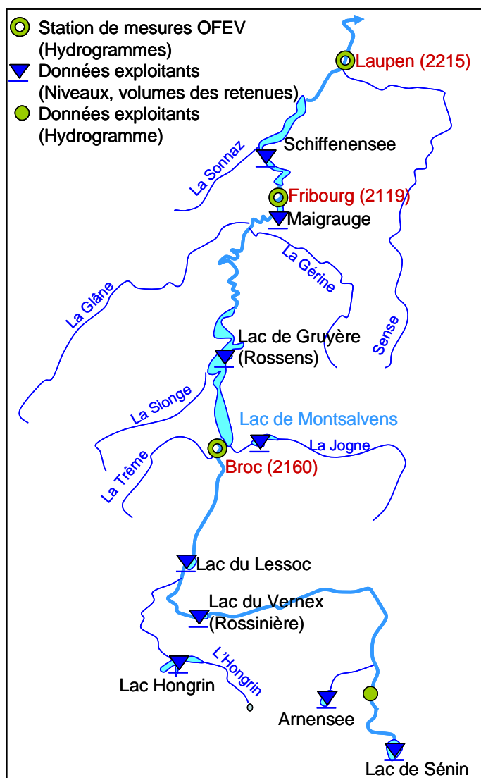
Figure 8 : Réseau hydrographique de la Sarine modélisé dans Routing System Localisation des points de calage
