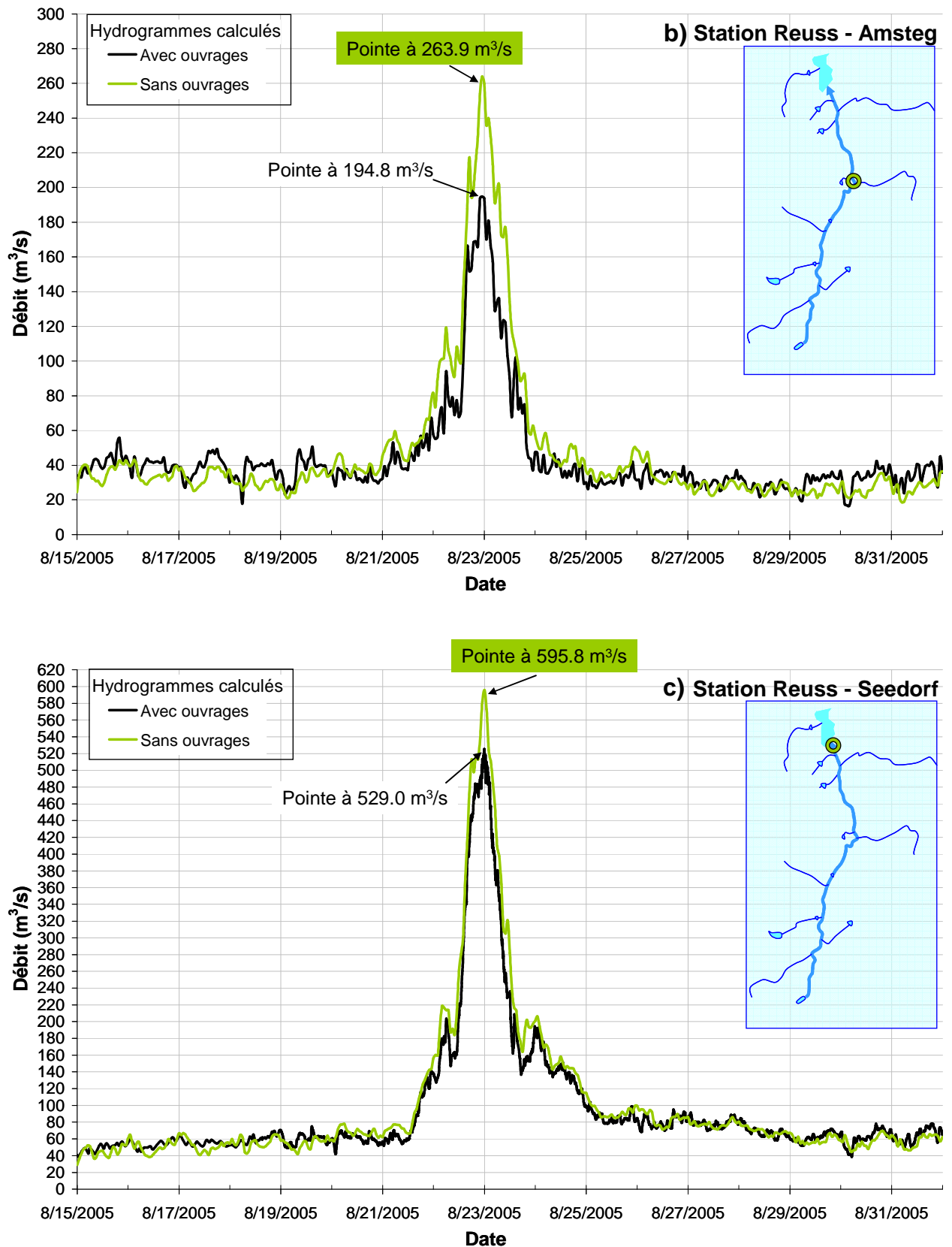
Figure 36 : Hydrogrammes actuels avec ouvrages (en noir) et naturel sans ouvrages (en vert) à la station d'Andermatt (a), à Amsteg (b) et à la station de Seedorf (c) sur la Reuss
