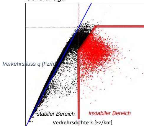
Abbildung 59 Fundamentaldiagramm für eine Zählstelle in eine Fahrrichtung
