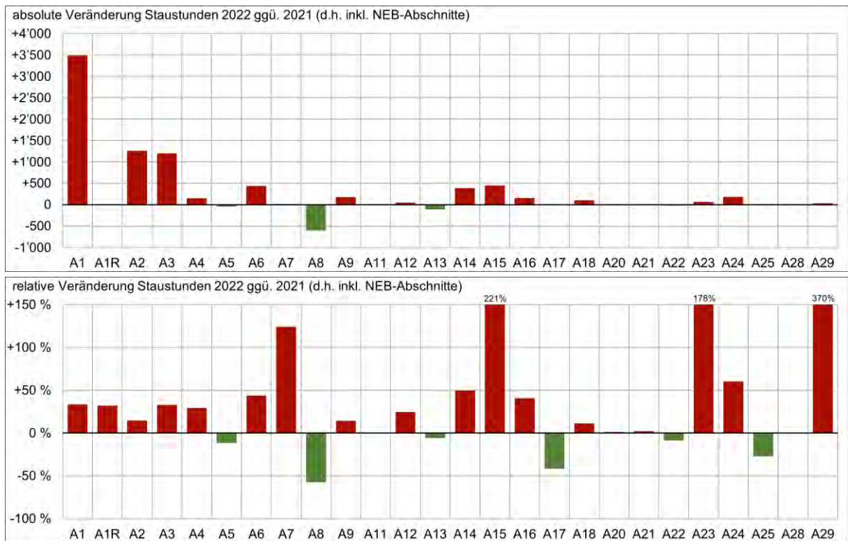
Abbildung 28: Veränderung der Staustunden 2022 gegenüber 2021 nach Nationalstrassen (inkl. NEB) Quellen: ASTRA: VMON, Viasuisse
