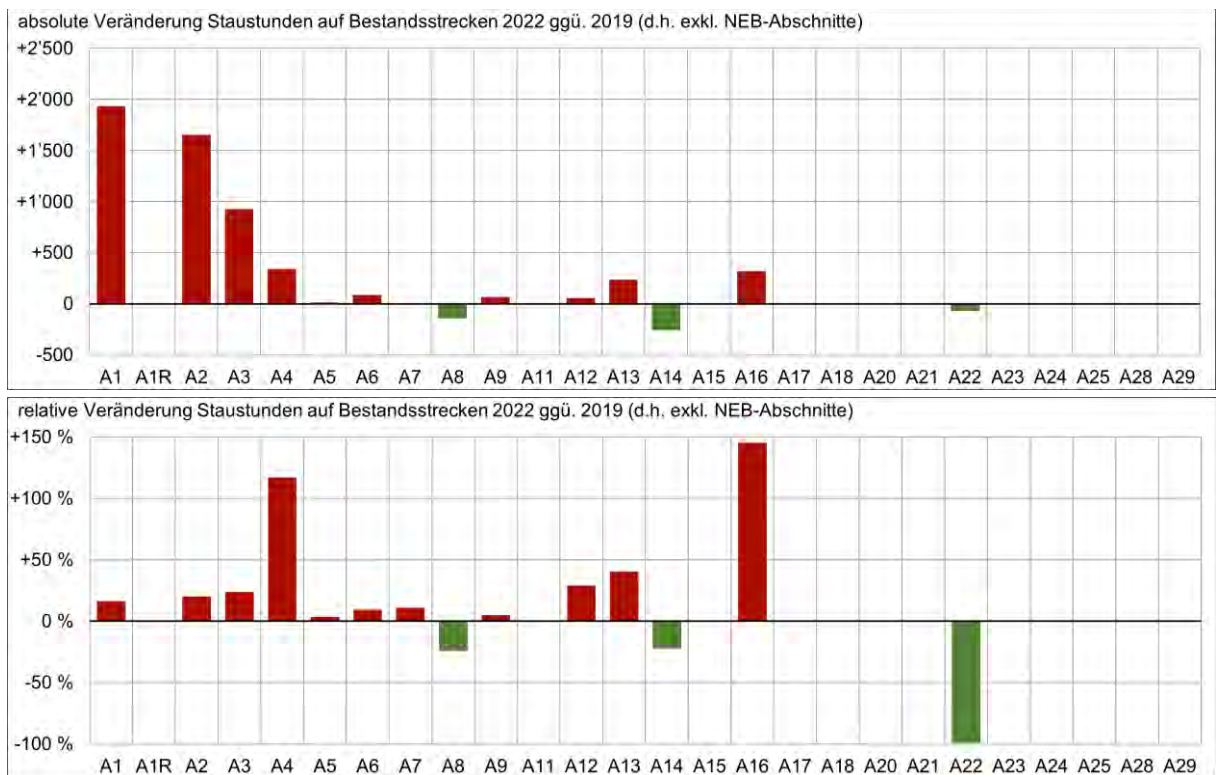
Abbildung 29: Veränderung der Staustunden 2022 gegenüber 2019 nach Bestandsstrecken Quellen: ASTRA: VMON, Viasuisse
