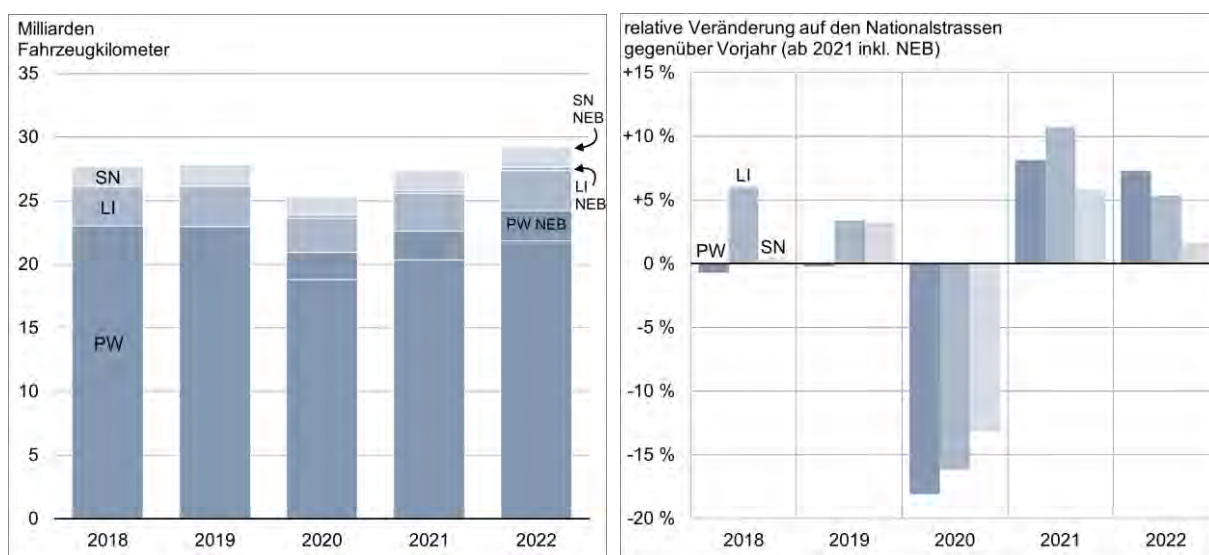
Abbildung 6: Verkehrsentwicklung auf dem Nationalstrassennetz nach Personen- und Güterverkehr
