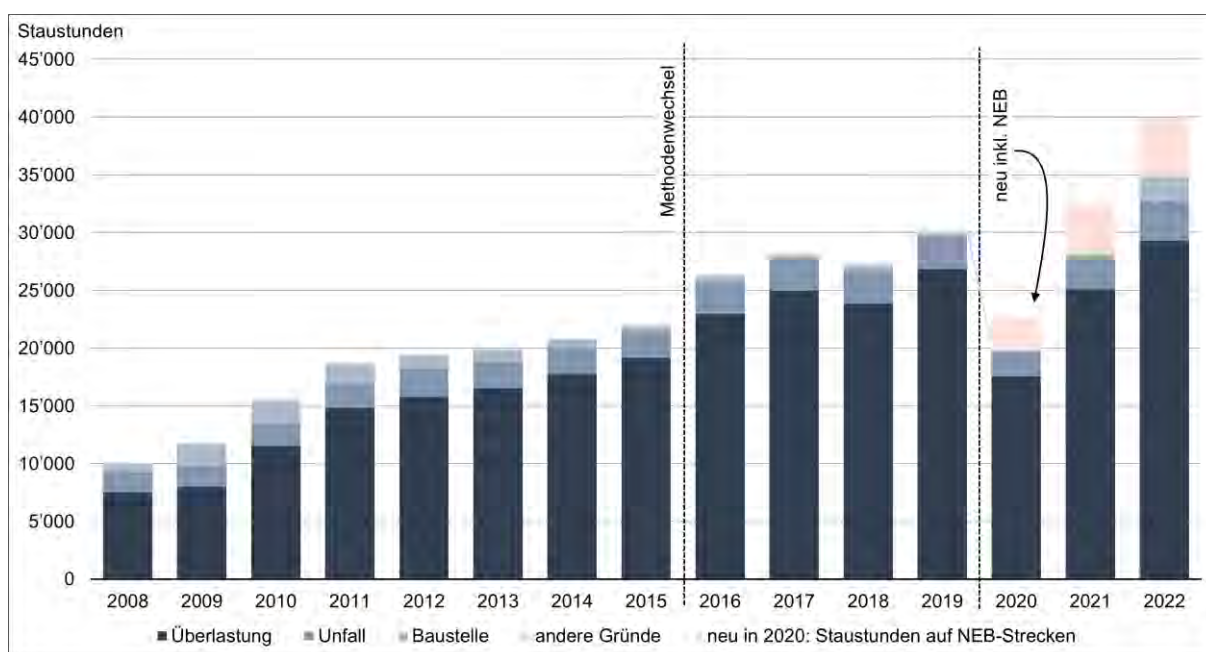
Abbildung 23: Entwicklung der Staustunden auf den Nationalstrassen Quellen: ASTRA: VMON, Viasuisse
