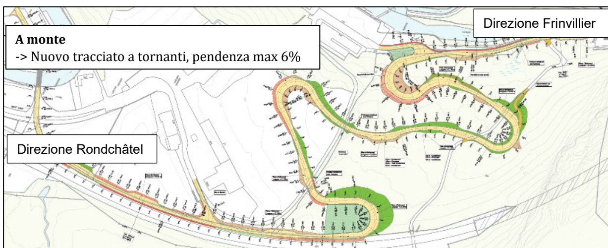
Il nuovo tracciato a tornanti
