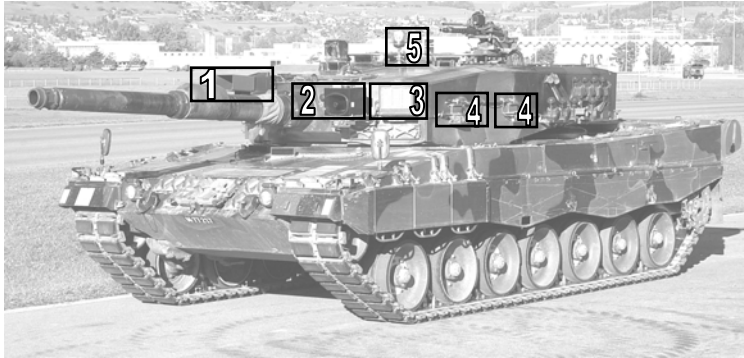
1 : émetteur laser ; 2 : haut-parleur actif ; 3 : appareil de visualisation 4 : réflecteurs / récepteurs ; 5 : feu tournant
