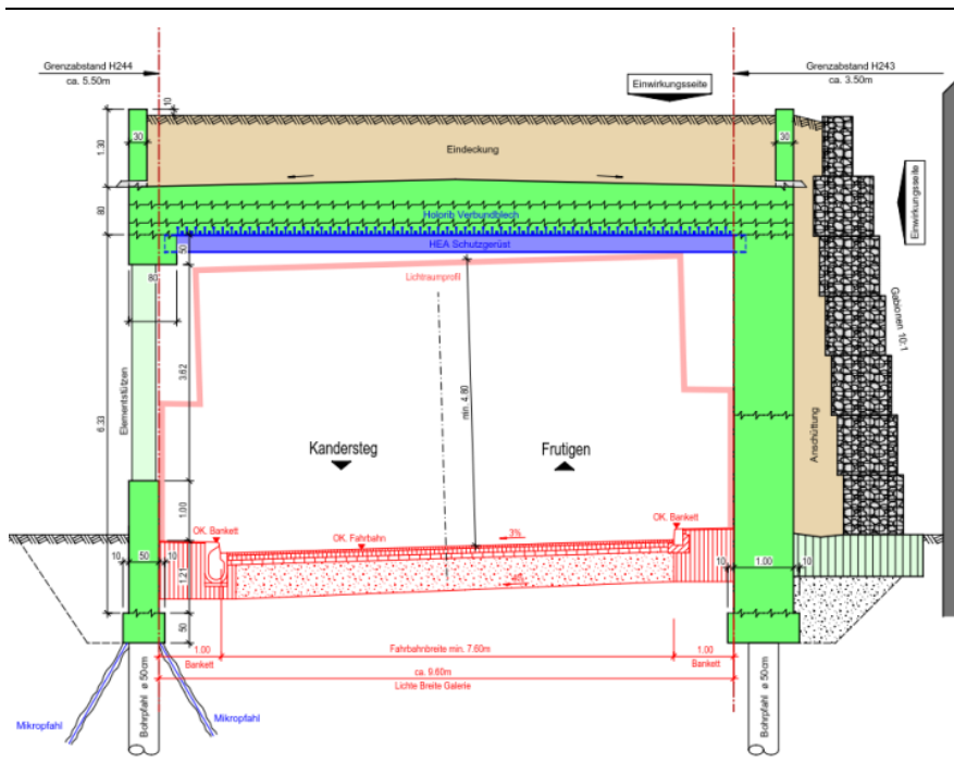
Abbildung 2: Normalprofil Variante a (Quelle: Synthesebericht Varianten, Heierli Ingenieurbau AG)
