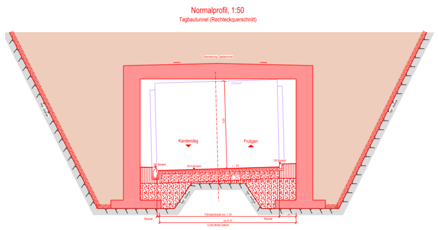
Abbildung 3: Normalprofil Variante b (Quelle: Synthesebericht Varianten, Heierli Ingenieurbau AG)
