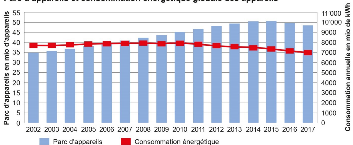
Graphique 1: Modifications du parc et évolution de la consommation électrique de tous les appareils recensés
