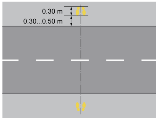
Fig. 8 Esempio di applicazione della demarcazione «piedini»
