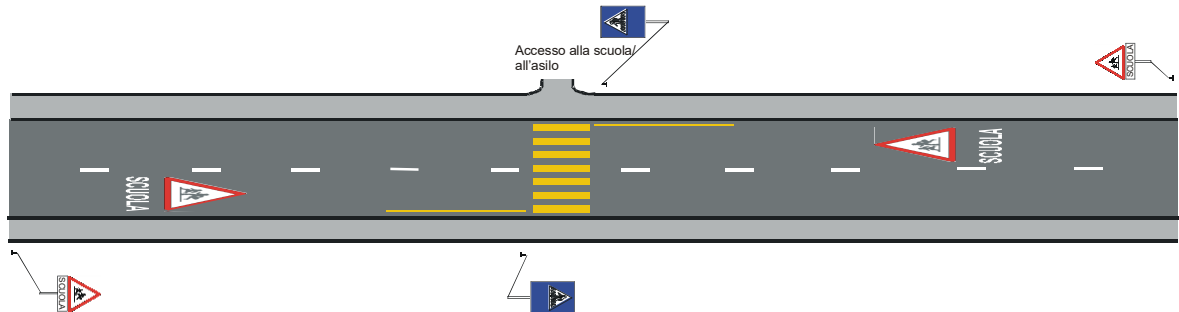
Fig. 1 Disposizione della demarcazione e del segnale di pericolo «Bambini» Esempio di un punto di attraversamento con strisce pedonali
