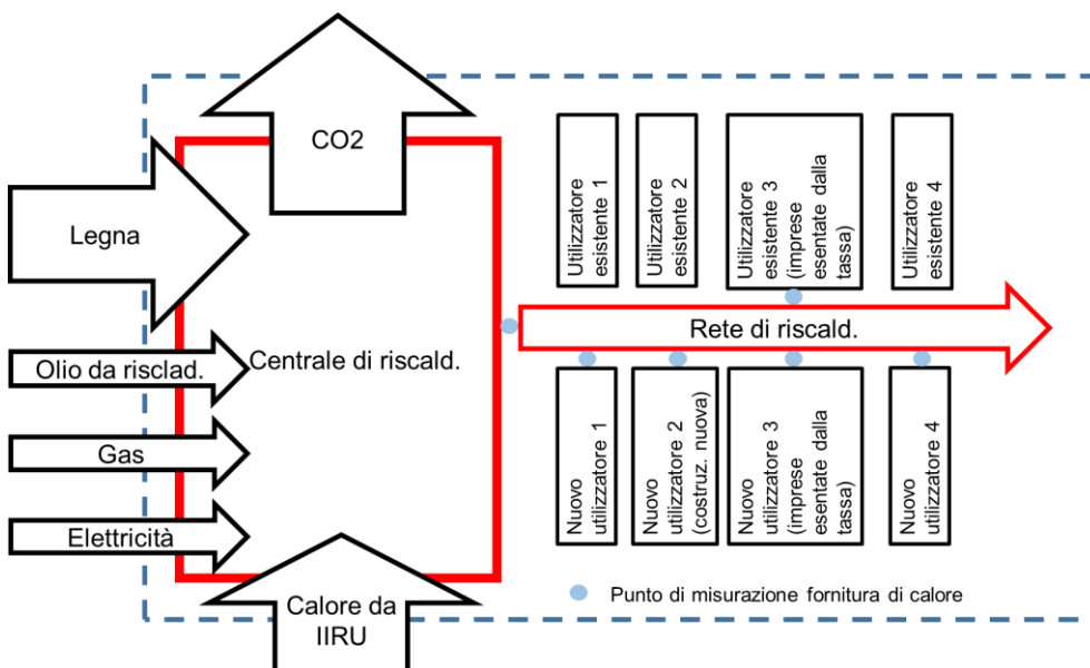
Figura 3: Limiti del sistema per il progetto o il progetto di un programma: tutte le fonti di calore della centrale di riscaldamento esistente e nuova nonché tutti gli utilizzatori di calore rientrano nei limiti del sistema
