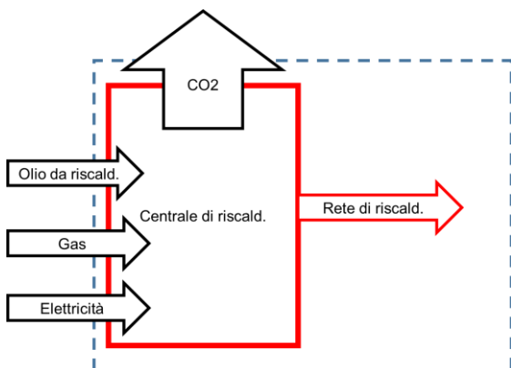
Figura 2: Limiti del sistema per lo scenario di riferimento in una rete di riscaldamento a distanza esistente: nel campo d'applicazione dell'ordinanza rientrano solo le reti di riscaldamento esistenti esclusivamente a combustibili fossili e quindi anche nello sviluppo di riferimento sarebbero ancora esclusivamente a combustibili fossili
