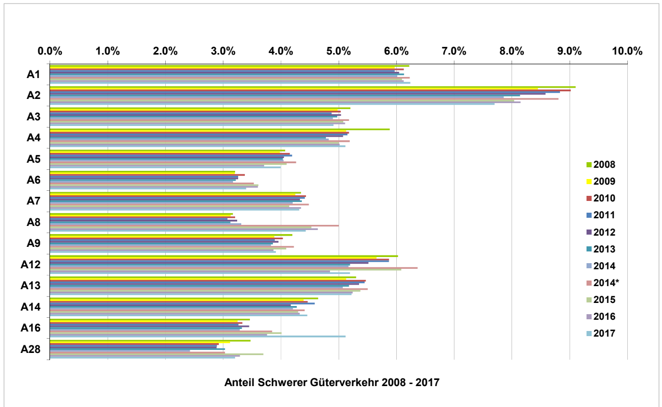
Abbildung 9 Anteil Schwerer Güterverkehr 2008-2017
