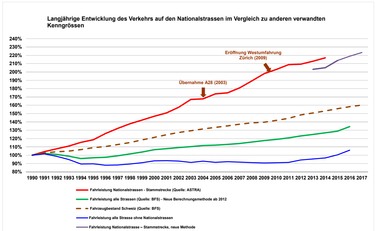
Abbildung 1 Entwicklung des Verkehrs auf den Nationalstrassen: Durchschnittlicher täglicher Verkehr
