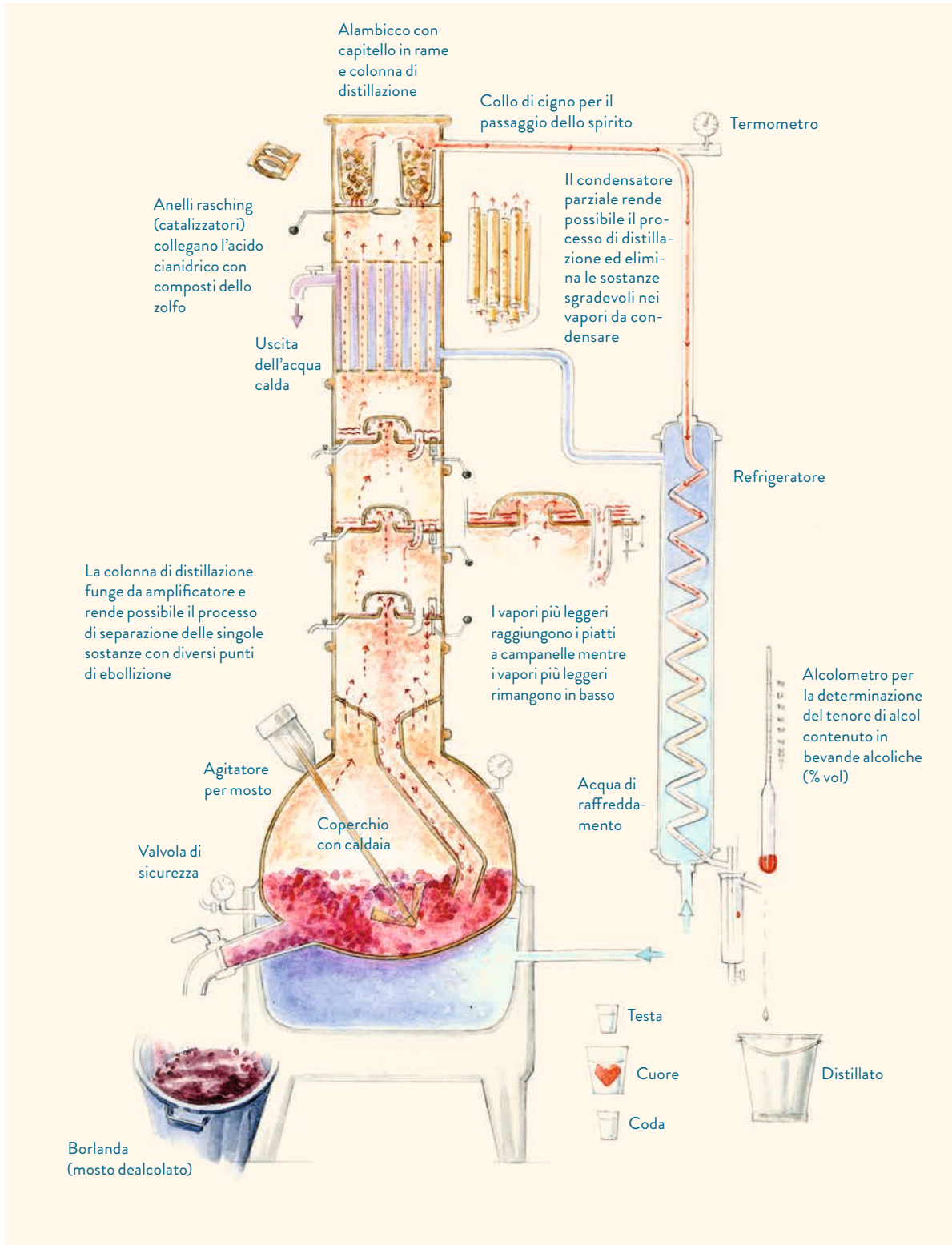
12 Impianto di distillazione e processo di distillazione.
