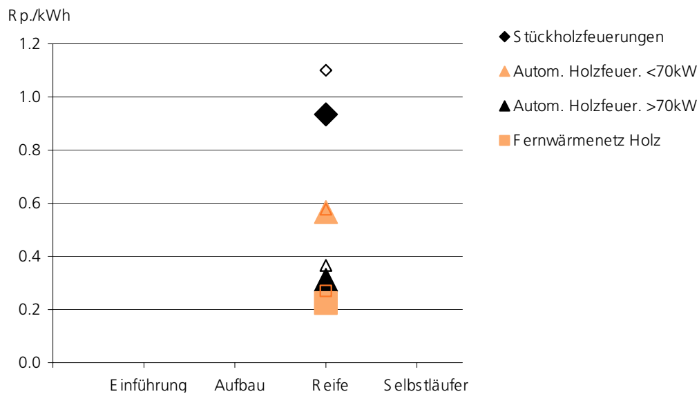
Figur 21: Kostenintensitäten von Massnahmen im Bereich Holzenergie für die Berichtsjahre 2004 und 2005. Die kleinen leeren Kästchen markieren den Wert für das Berichtsjahr 2004, volle für 2005.
