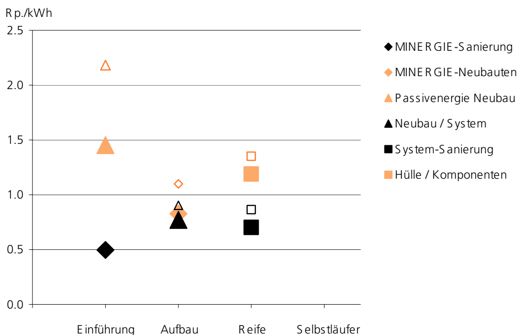
Figur 19: Kostenintensität von Massnahmen im Energieeffizienzbereich für die Berichtsjahre 2004 und 2005. Die kleinen leeren Kästchen markieren den Wert für das Berichtsjahr 2004, volle für 2005.
