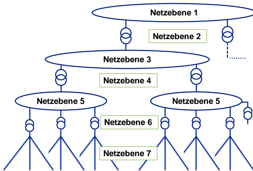
Abbildung 21: Netzebenen
