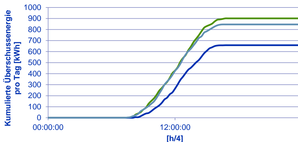
Abbildung 26: Kumulierte Energiemenge für ausgewählte Überlastungsereignisse
