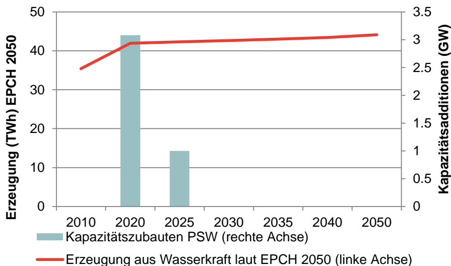
Abbildung 23. Entwicklung der Wasserkrafterzeugung laut EPCH 2050 und geplante PSW-Zubauten
