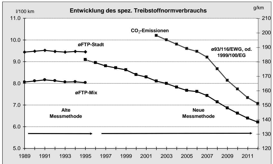
Grafik 1 Spezifischer Treibstoffnormverbrauch seit 1989
