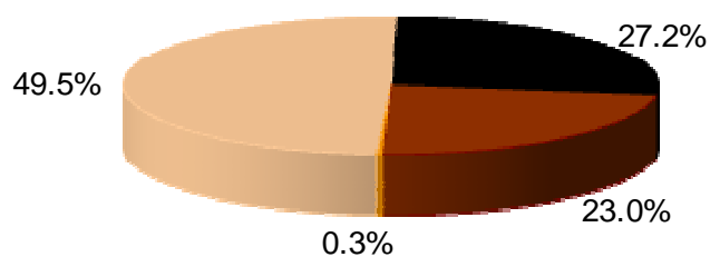
Grafik 3: Prozentuale Verteilung der CO 2 -Emissionen aus Brennstoffen (klimakorrigiert), Jahr 2011
