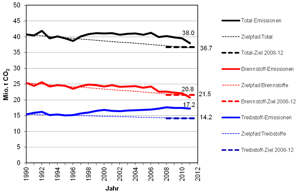
Grafik 2: Entwicklung der CO 2 -Emissionen gemäss CO 2 -Gesetz (Zeitreihe 1990 – 2011), Angaben in Millionen Tonnen CO 2 . Die dünnen Linien markieren den jeweiligen Zielpfad, ohne Berücksichtigung des Erwerbs von ausländischen CO 2 -Zertifikaten. Die Emissionswerte der Brennstoffe sind klimakorrigiert.
