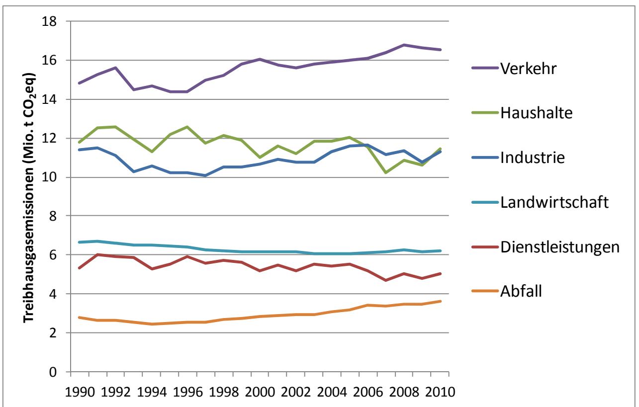
Abb. 1: Entwicklung der Treibhausgasemissionen 1990 – 2010 in Millionen Tonnen CO 2 -Äquivalenten
