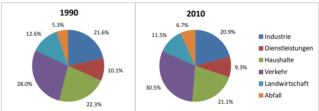
Abb. 2: Anteile der einzelnen Sektoren an den Treibhausgasemission der Jahre 1990 und 2010
