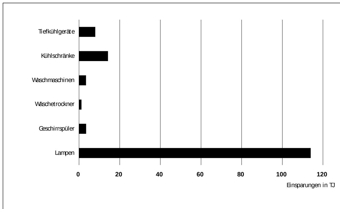
Figur 18: Abschätzung der Einsparungen aufgrund der Energieetikette bei den 2003 neu verkauften Haushaltgeräte und Lampen in TJ pro Jahr (Quelle: Schätzung INFRAS auf der Grundlage der Marktdaten eae/FEA und der eae/SLG sowie der Schätzungen der Discrete Choice Analyse im Kapitel 3.3.2).
