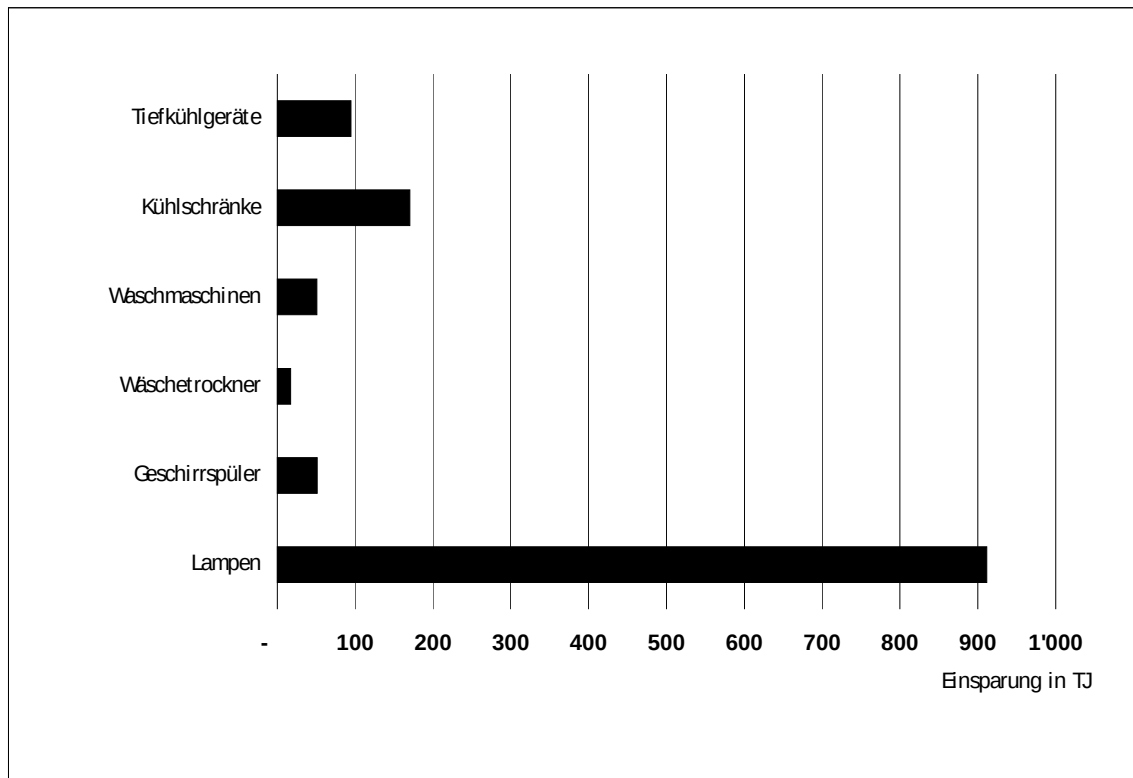
Figur 21: Abschätzung der Einsparungen aufgrund der Energieetikette bei den 2003 neu verkauften Haushaltgeräte und Lampen über die Lebensdauer (Quelle: Schätzung INFRAS auf der Grundlage der Marktdaten eae/FEA und der eae/SLG sowie der Schätzungen der Discrete Choice Analyse im Kapitel 3.3.2).
