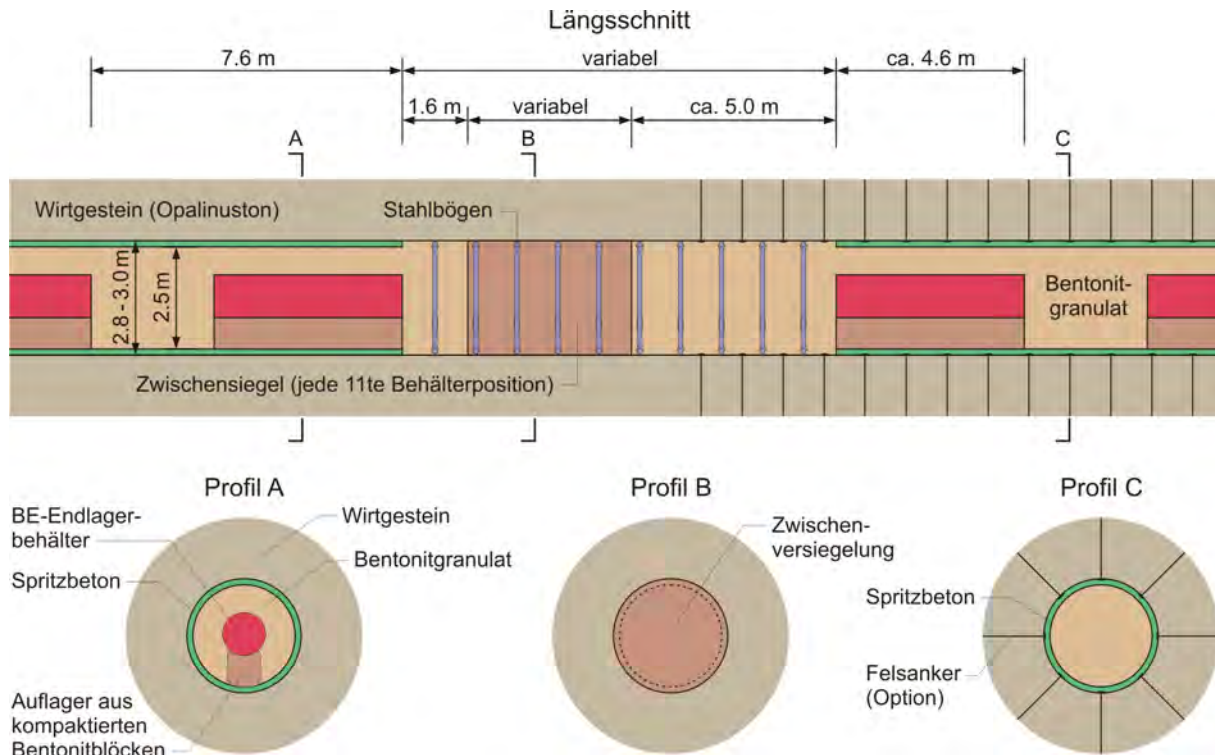
Figur 8-1: Konzept für den Ausbau der HAA-Lagerstollen mittels Spritzbeton (NTB 10-01, S. 122).
