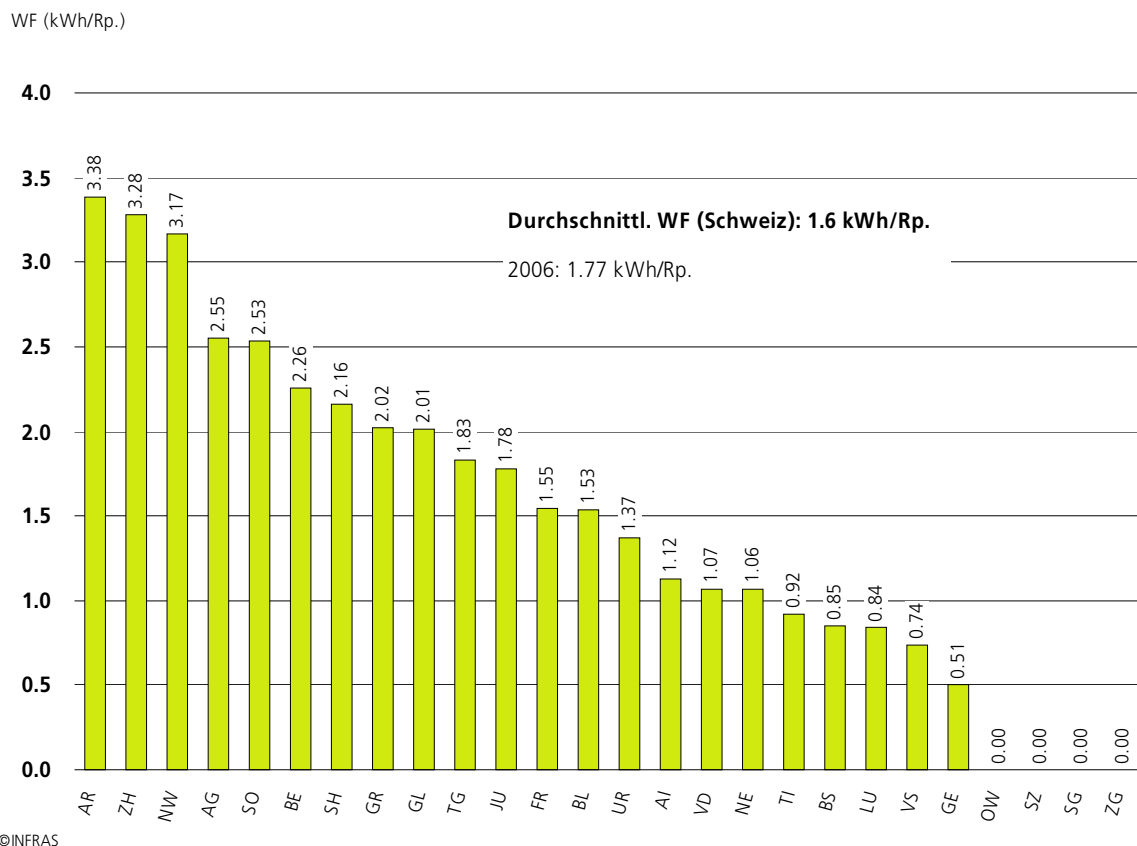
Figur 13: Wirkungsfaktoren 2007 nach Kantonen.
