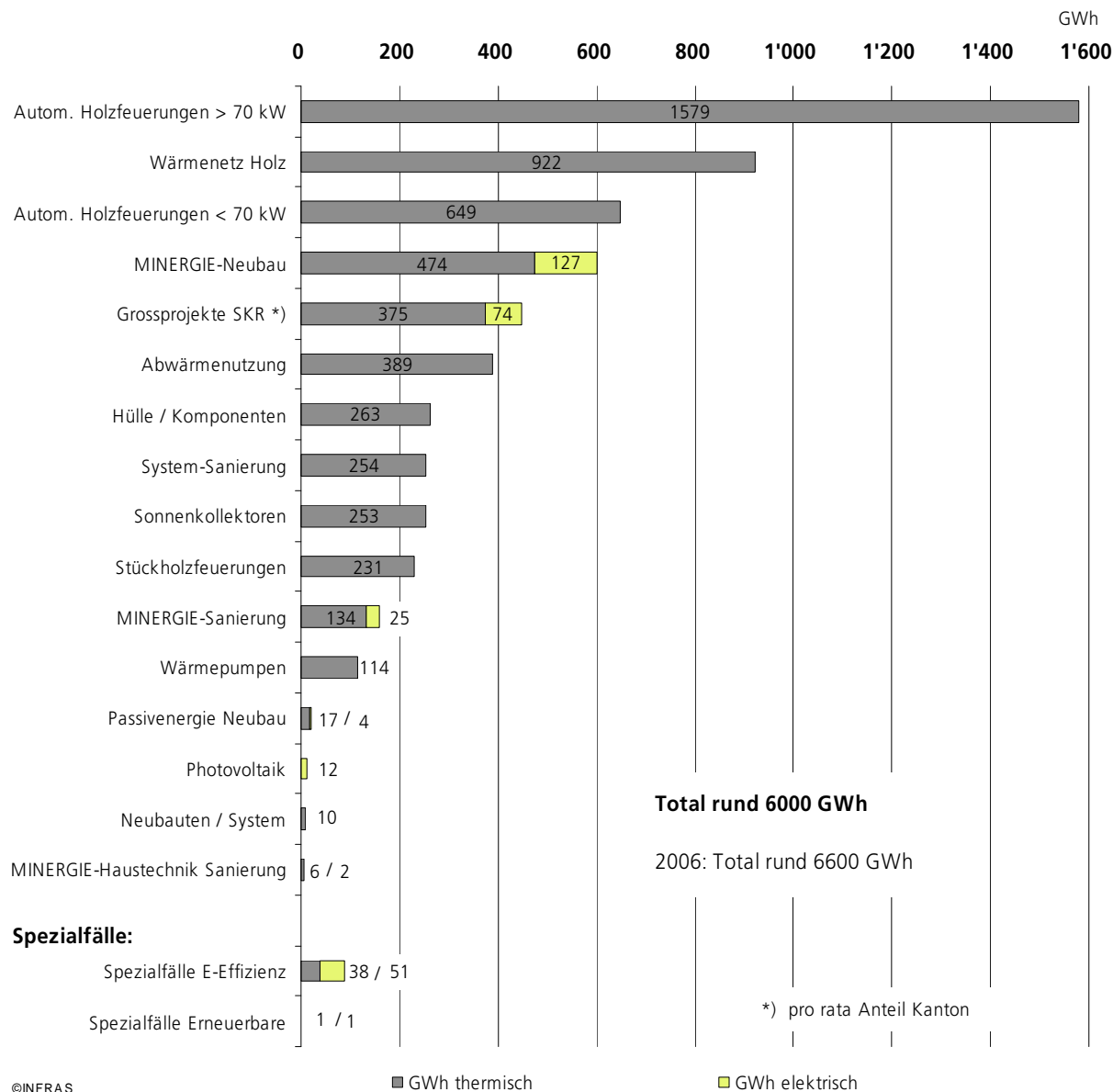
Figur 4: Energetische Wirkungen der kantonalen Förderprogramme im Jahr 2007 (direkte Massnahmen über Lebensdauer).
